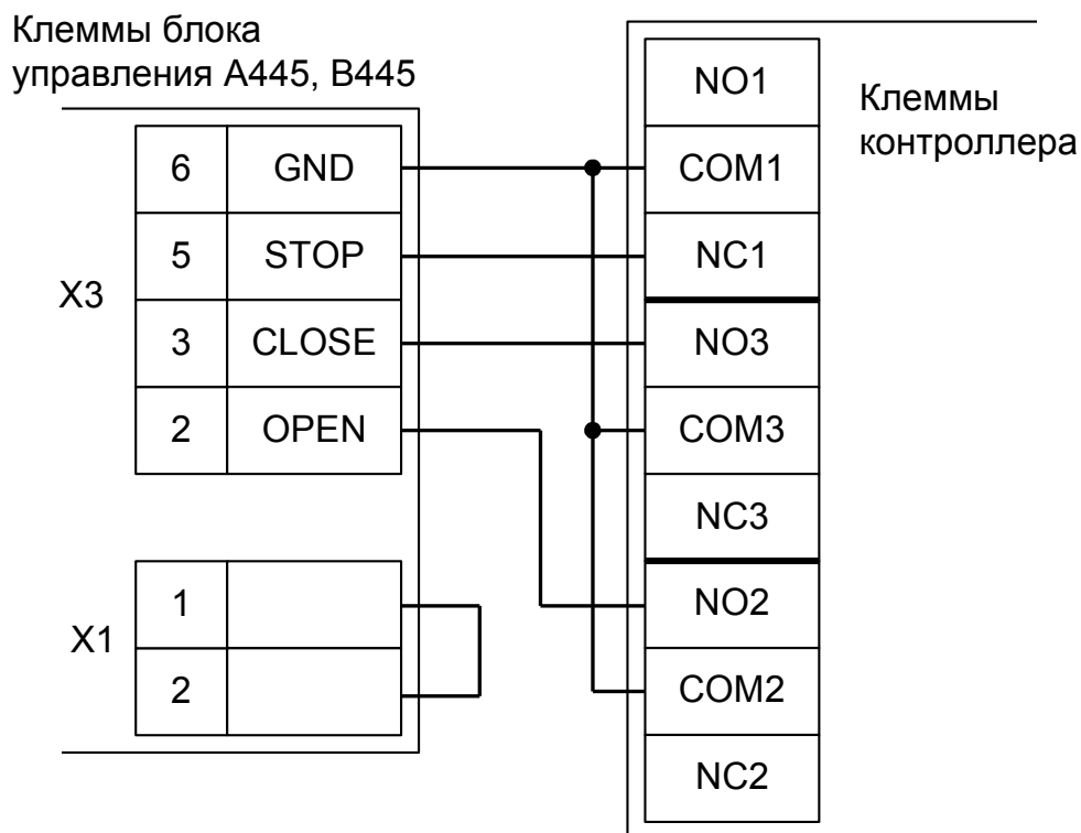
Рисунок 145. Подключение блоков управления Normann A445, B445.
