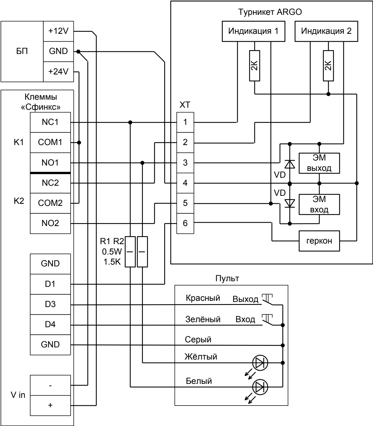
Рисунок 99. Подключение турникета ARGO.
