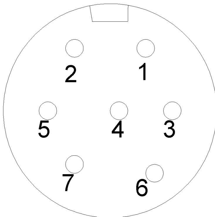
Рисунок 51. Разъём PC7.
