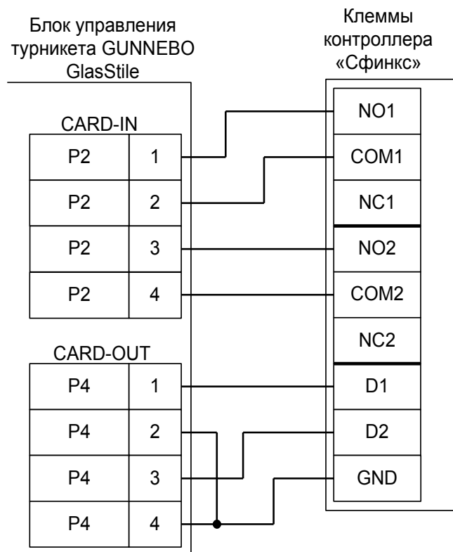
Рисунок 92. Подключение турникета GlasStile.
