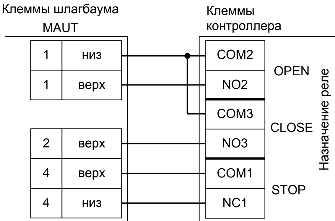
Рисунок 159. Подключение ELKA MAUT 20-35.
