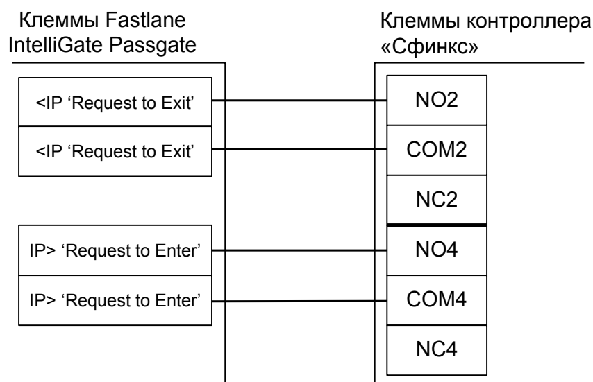
Рисунок 100. Подключение калитки Fastlane IntelliGate Passgate.
