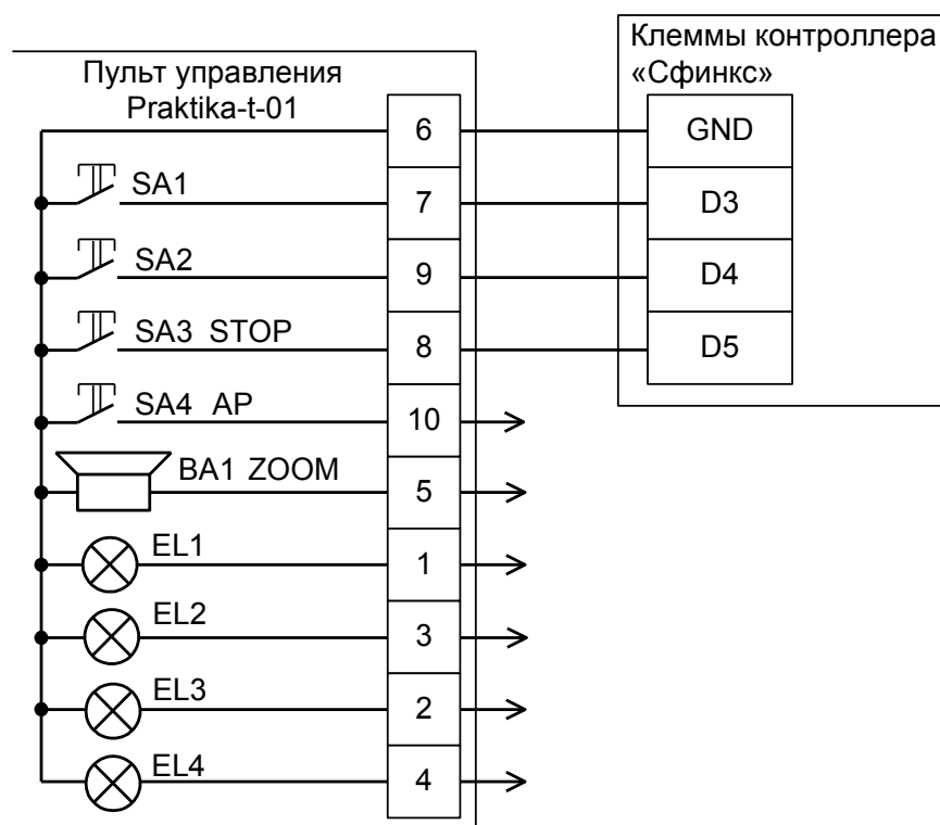
Рисунок 90. Подключение пульта управления Praktika.
