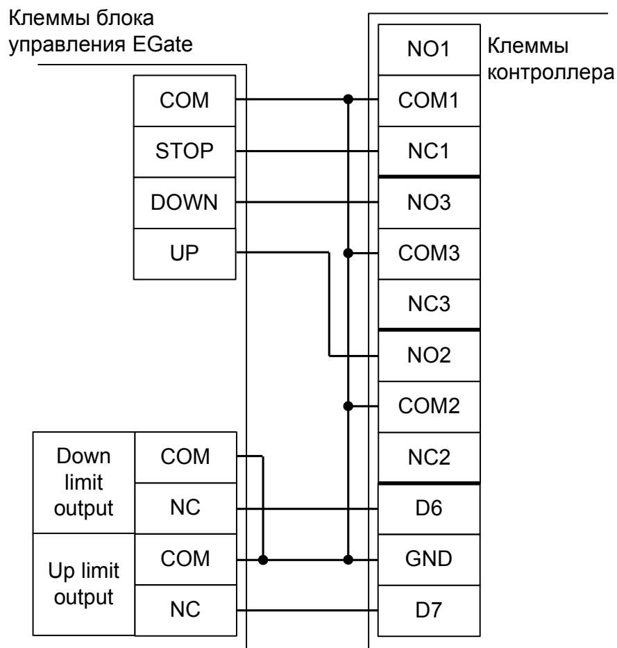
Рисунок 157. Подключение блока управления EGate.
