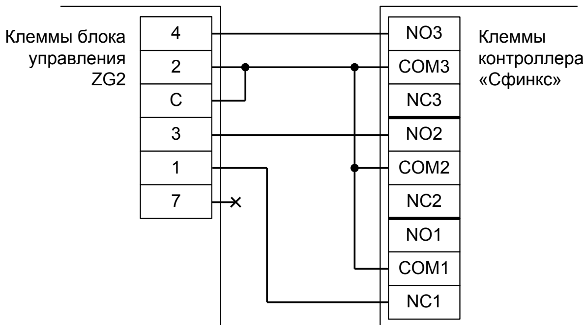
Рисунок 127. Подключение к блоку управления ZG2.
