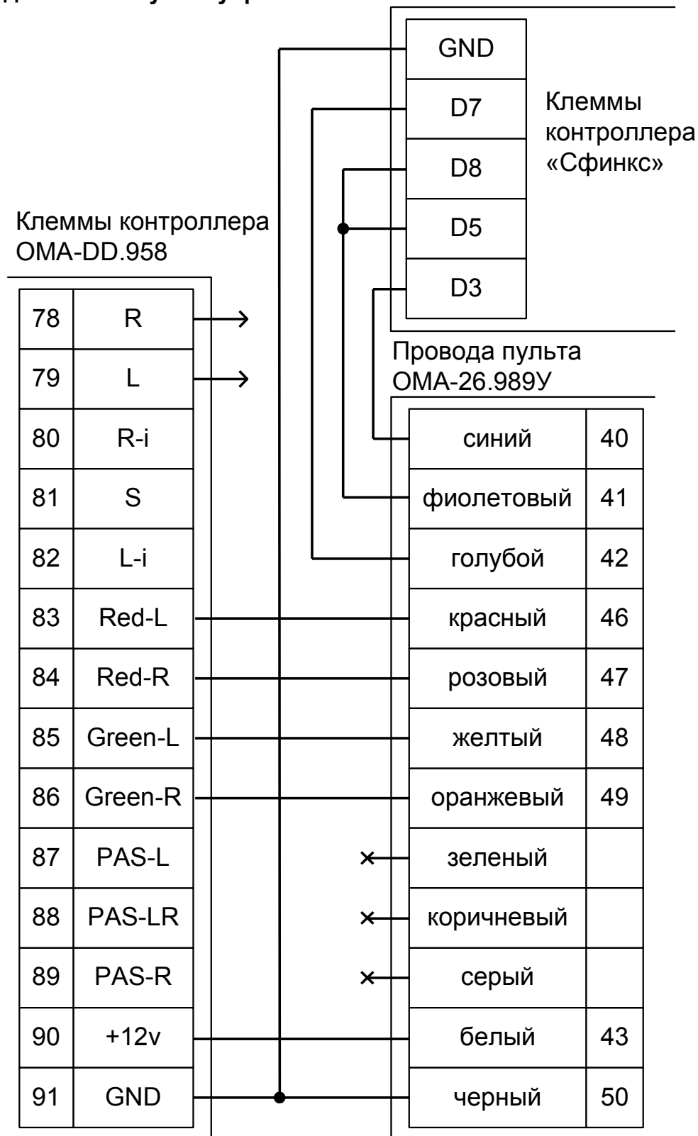
Рисунок 72. Подключение пульта управления калиткой ОМА-26.989У.
