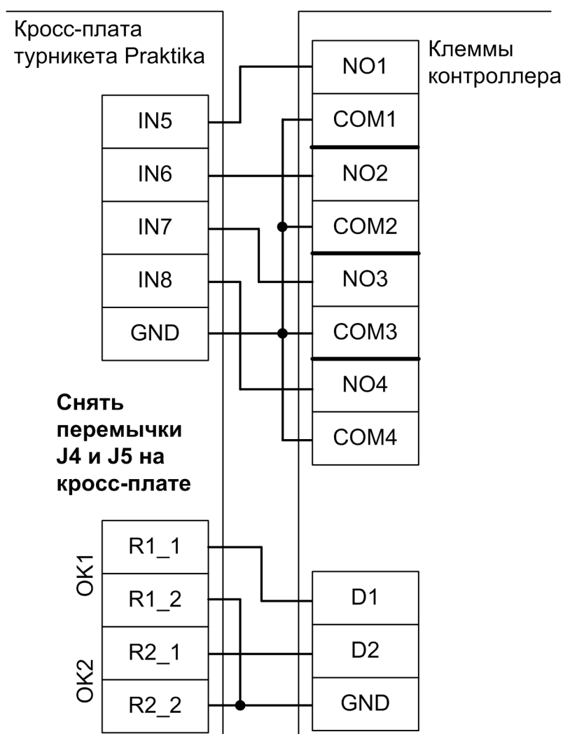
Рисунок 88. Подключение турникетов Praktika, старая электроника 1.
