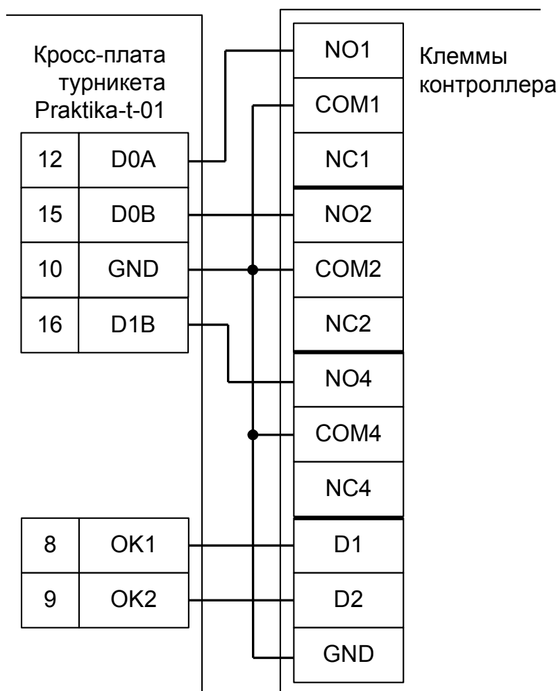
Рисунок 89. Подключение турникетов Praktika, старая электроника 2.
