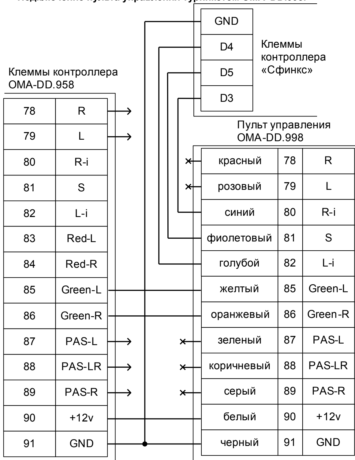
Рисунок 70. Подключение пульта управления турникетом ОМА–DD.998.
