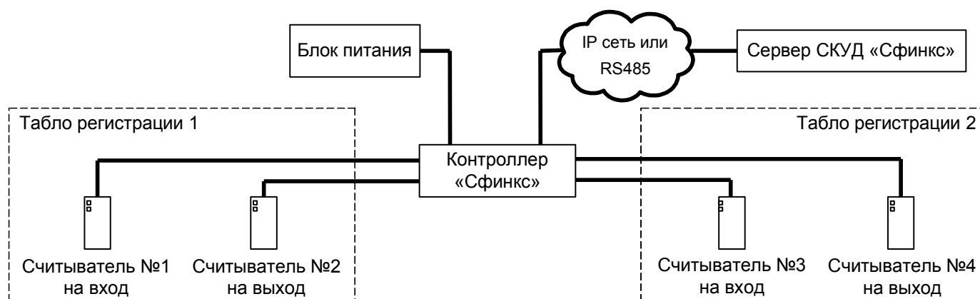
Рисунок 16. Вариант подключения в конфигурации «Терминал учёта рабочего времени».
