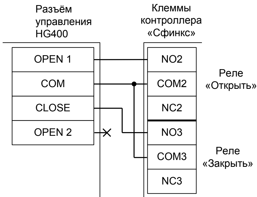
Рисунок 143. Подключение к шлагбауму Штрих-М HG400.
