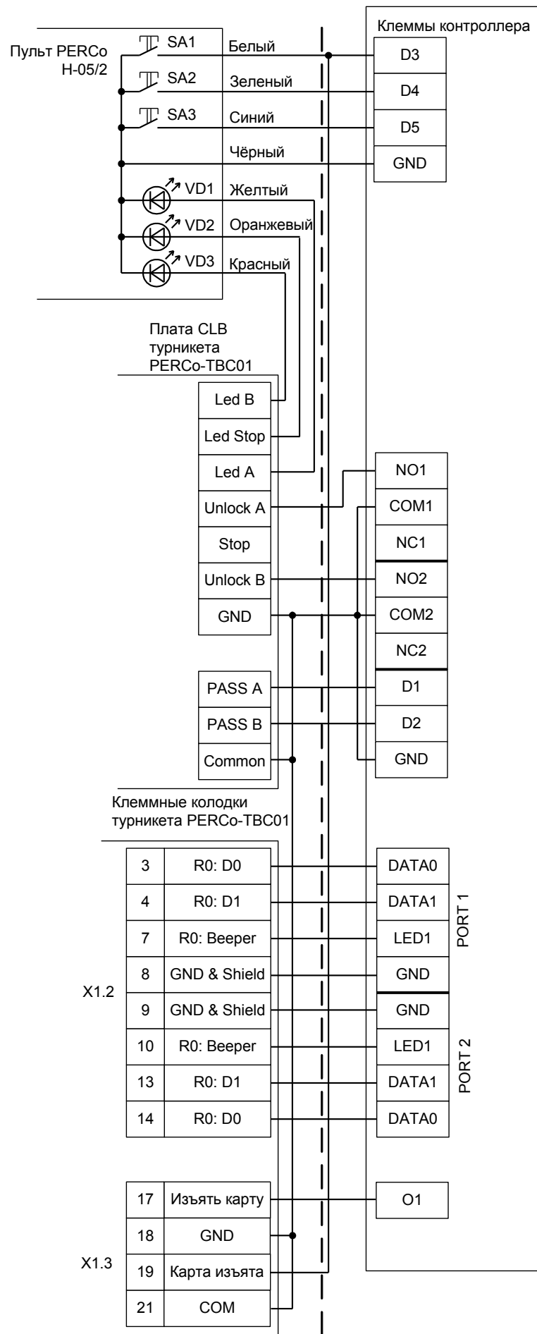
Рисунок 54. Подключение турникета PERCo-TBC01.
