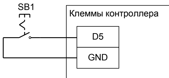
Рисунок 27. Подключение кнопки блокировки на примере первой двери.
