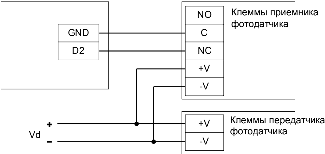
Рисунок 113. Подключение фотодатчика типа DOC на примере центрального датчика.
