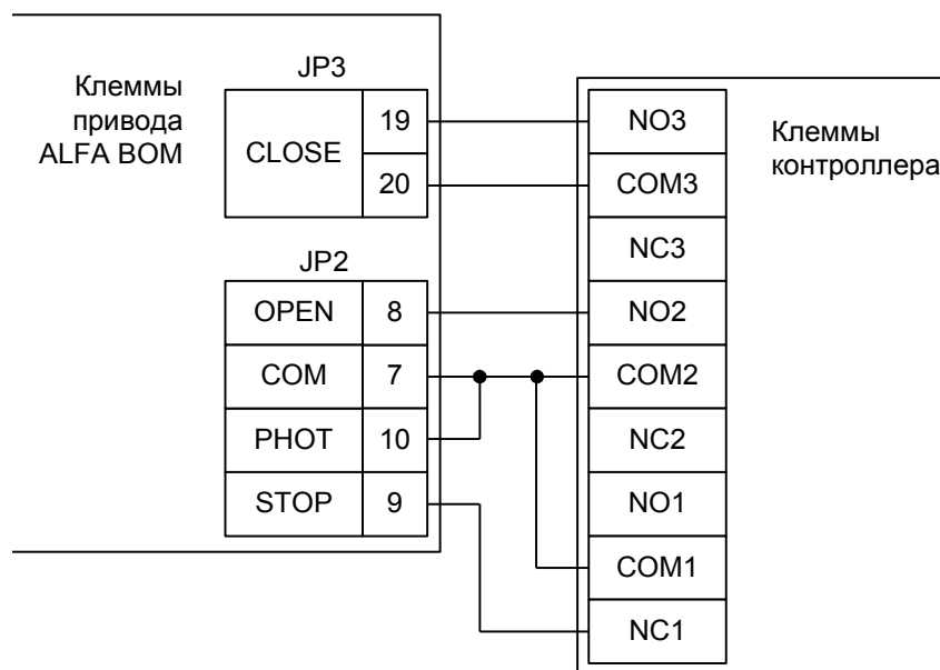
Рисунок 137. Подключение блока управления ALFA-BOM.
