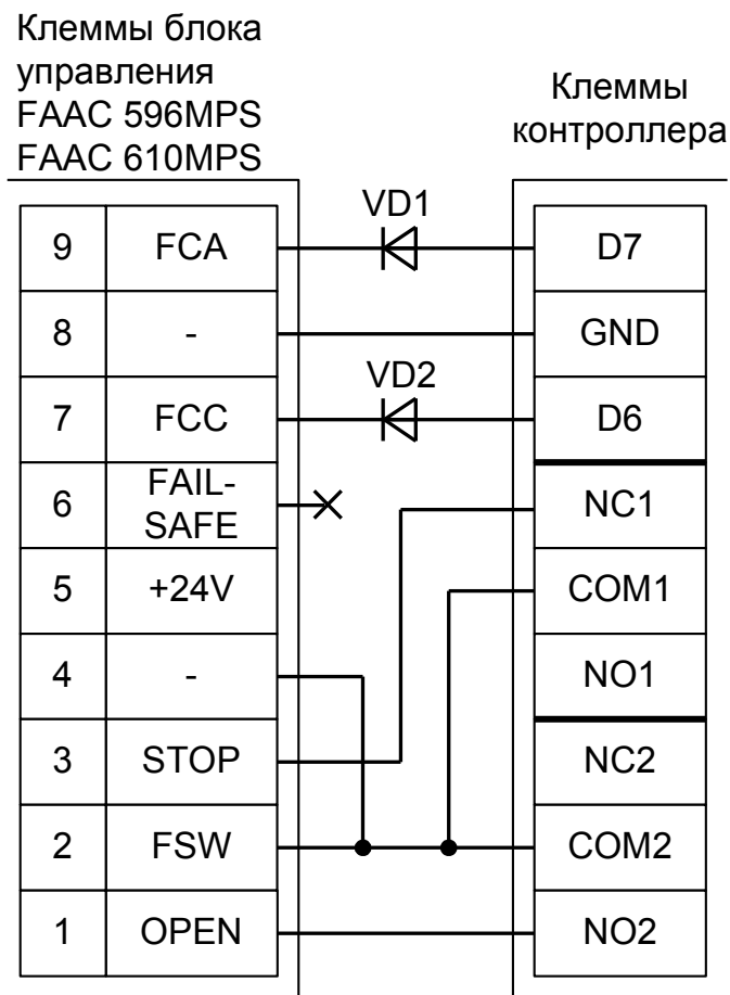
Рисунок 116. Подключение блока управления шлагбаумов FAAC 596MPS, FAAC 610MPS.
