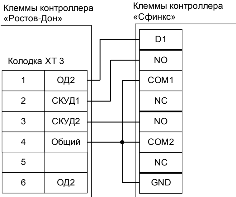
Рисунок 77. Подключение турникетов и калиток «Ростов–Дон», старая электроника, вариант №2.
