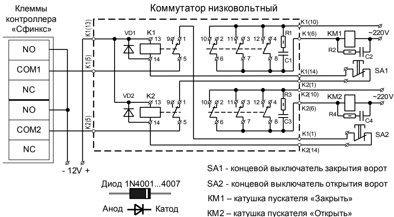
Рисунок 144. Пример подключения к приводу ворот, управляемому двумя электромагнитными пускателями.
