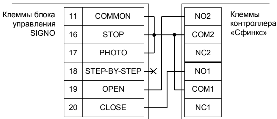
Рисунок 122. Подключение блока управления шлагбаумов SIGNO.
