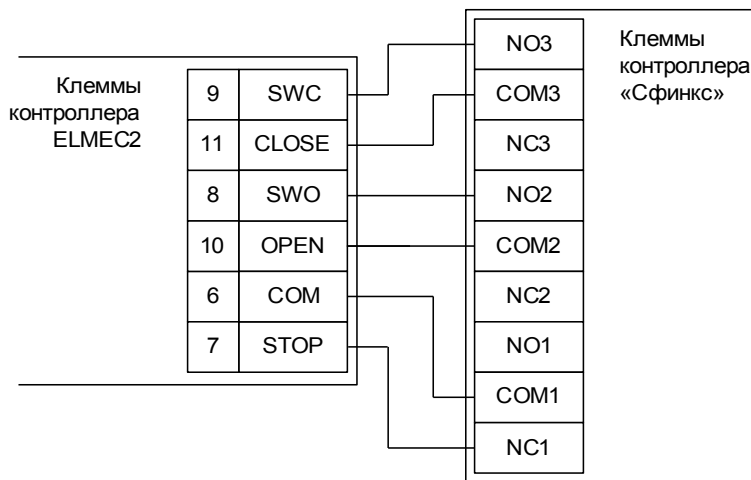
Рисунок 135. Подключение блока управления ELMEC1.
