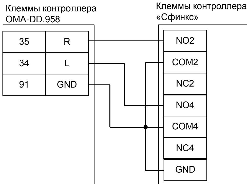
Рисунок 71. Подключение калитки ОМА 36.68 с контроллером ОМА-DD.958.
