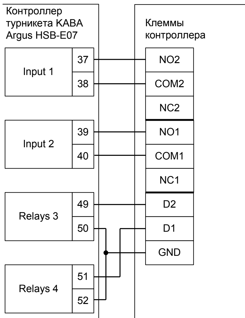
Рисунок 104. Подключение турникета KABA Argus HSB-E07 с платой управления ETS21.
