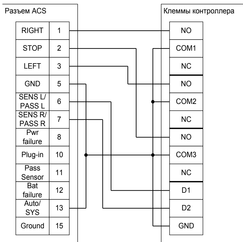
Рисунок 47. Подключение турникетов PERCo-TTR-04N и TTR-04W.
