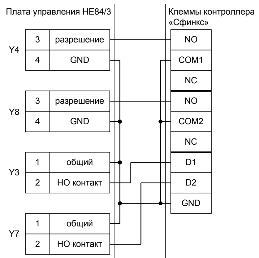
Рисунок 93. Подключение турникетов Gunnebo с платой управления HE84/3.
