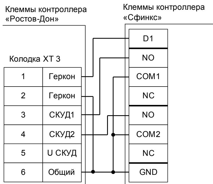
Рисунок 78. Подключение турникетов и калиток «Ростов–Дон», старая электроника, вариант №3.
