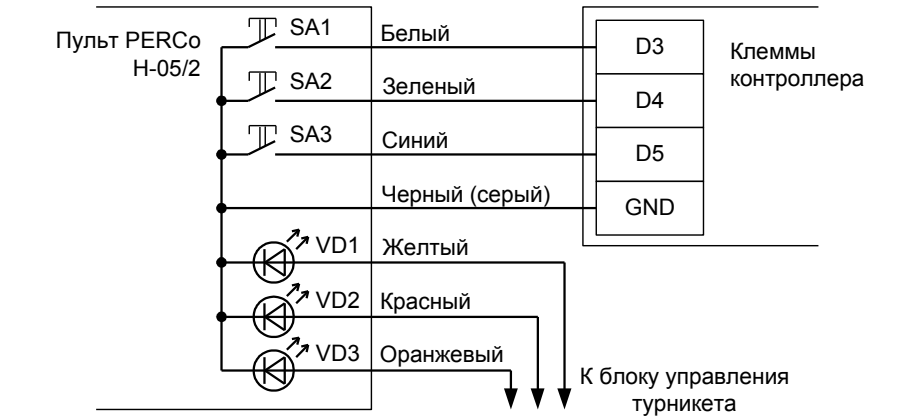
Рисунок 60. Подключение пульта управления PERCo H-05/2 без разъёма.
