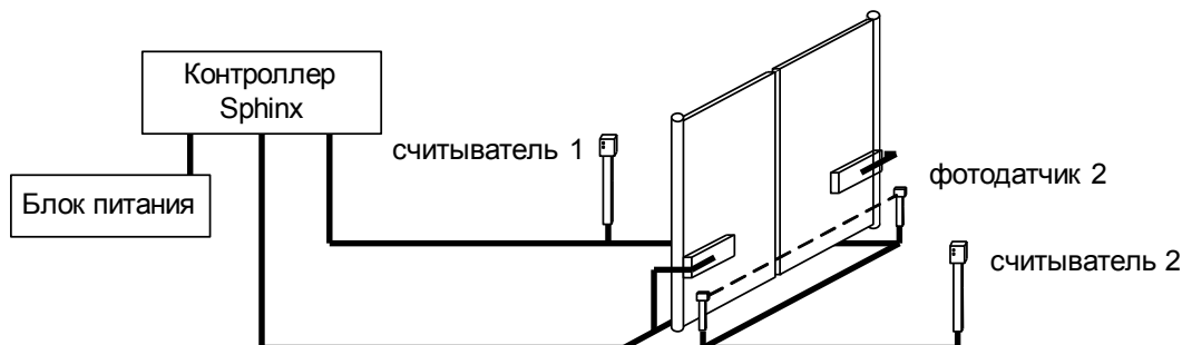
Рисунок 110. Пример автоматизации ворот с использованием прокси-карт или меток.
