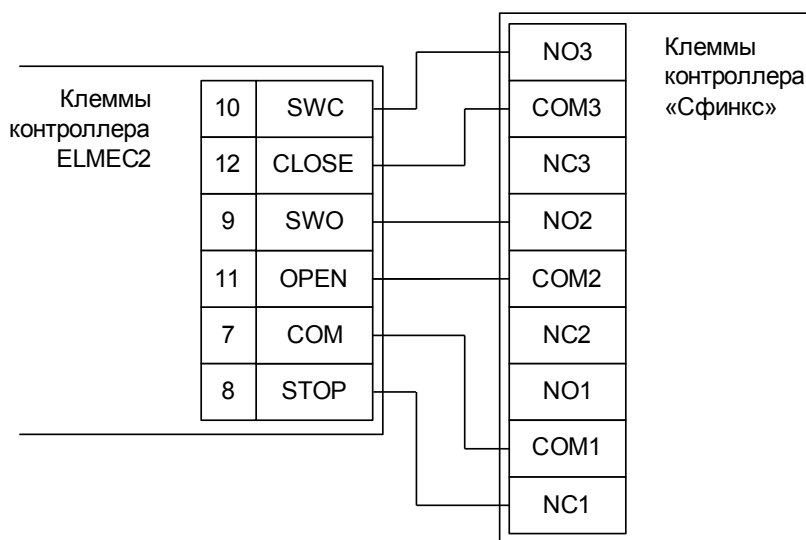
Рисунок 136. Подключение блока управления ELMEC2.
