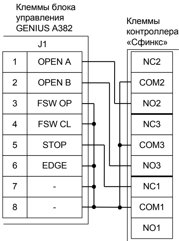
Рисунок 141. Подключение к блоку управления A382.
