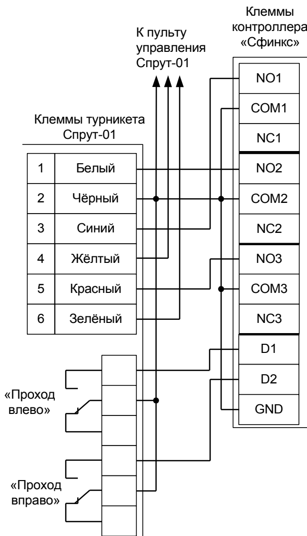
Рисунок 101. Подключение турникета «Спрут-01».
