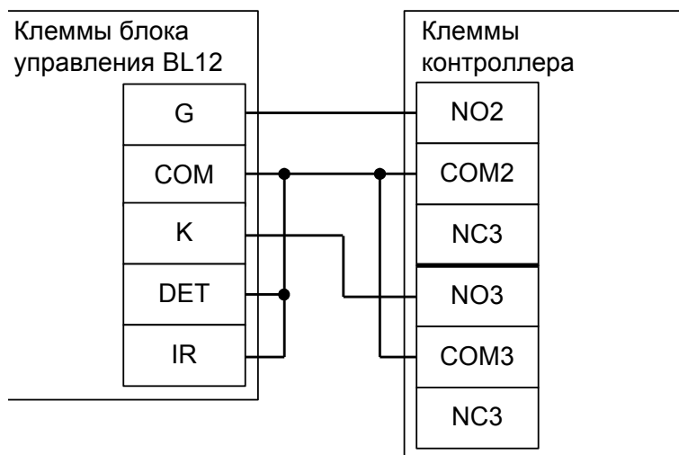
Рисунок 152. Подключение блока управления BL12.
