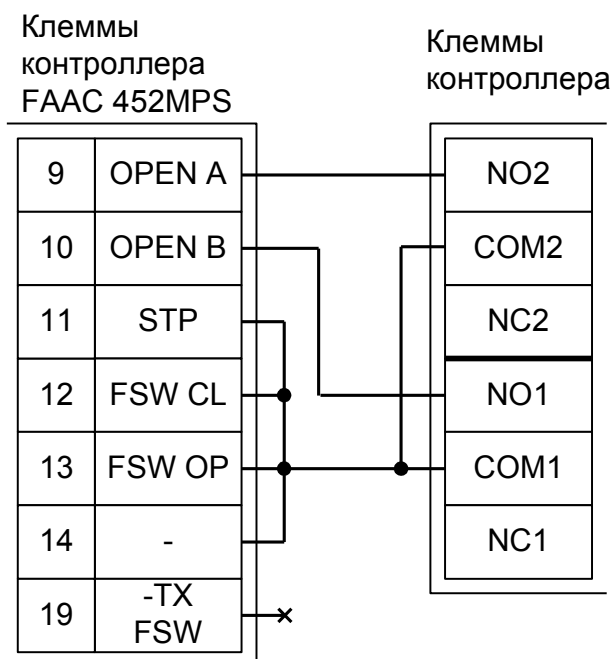
Рисунок 118. Подключение блока управления ворот FAAC 452MPS.
