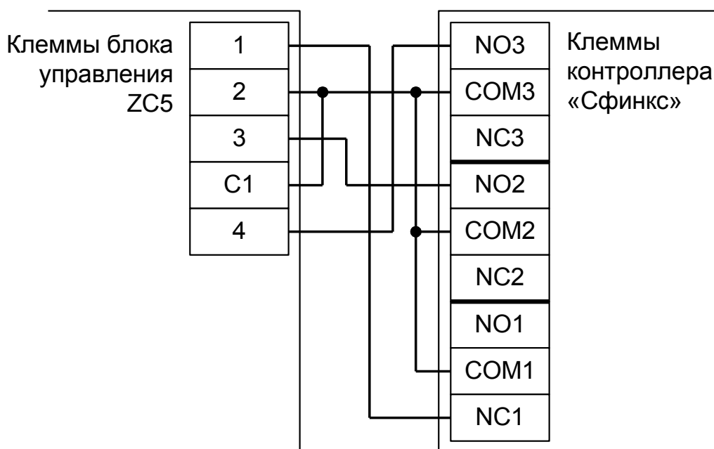
Рисунок 131. Подключение к блоку управления ZC5.
