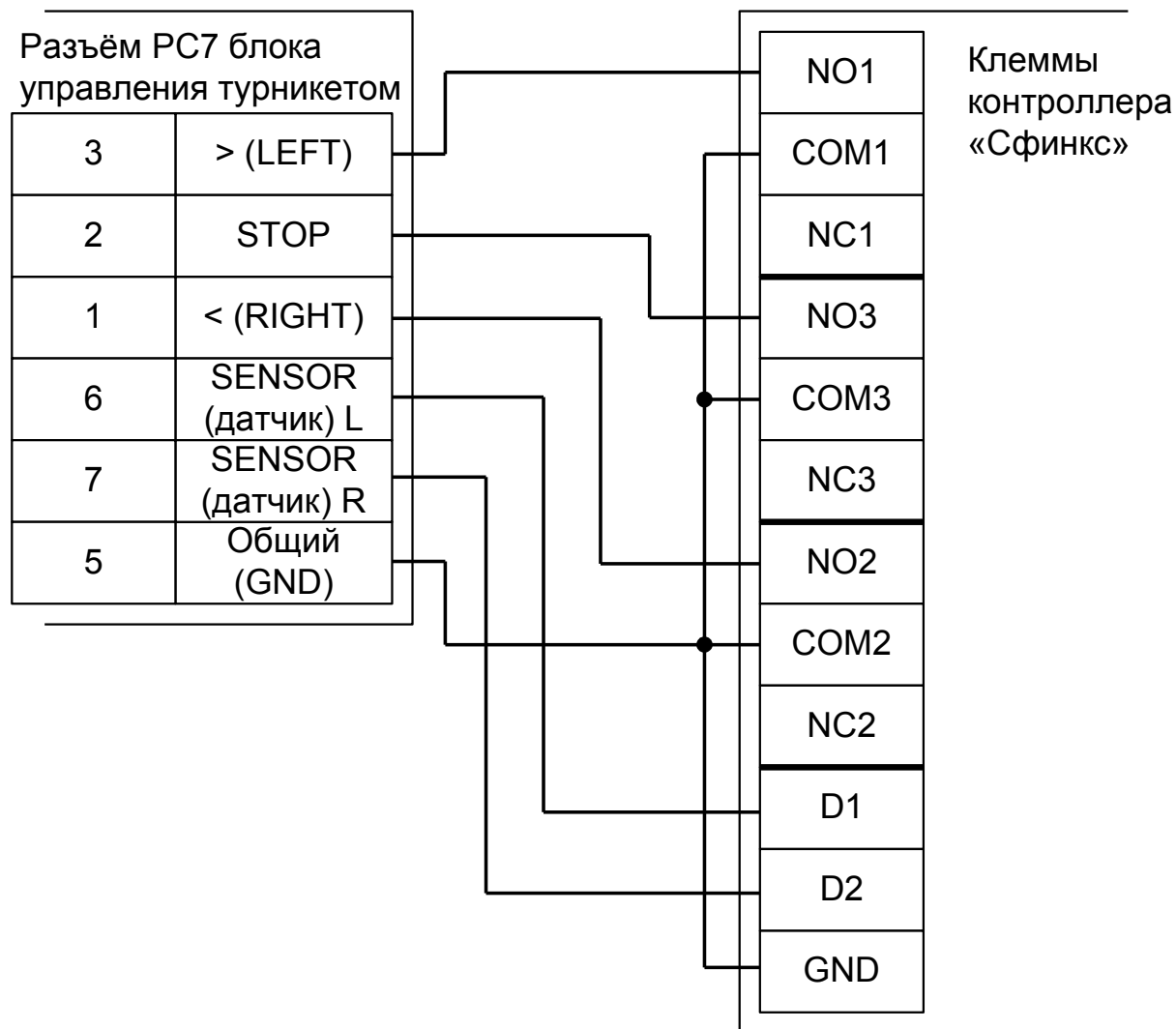
Рисунок 50. Подключение турникета PERCo-TTR-04.
