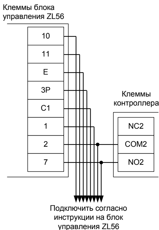
Рисунок 134. Подключение к блоку управления ZL56.
