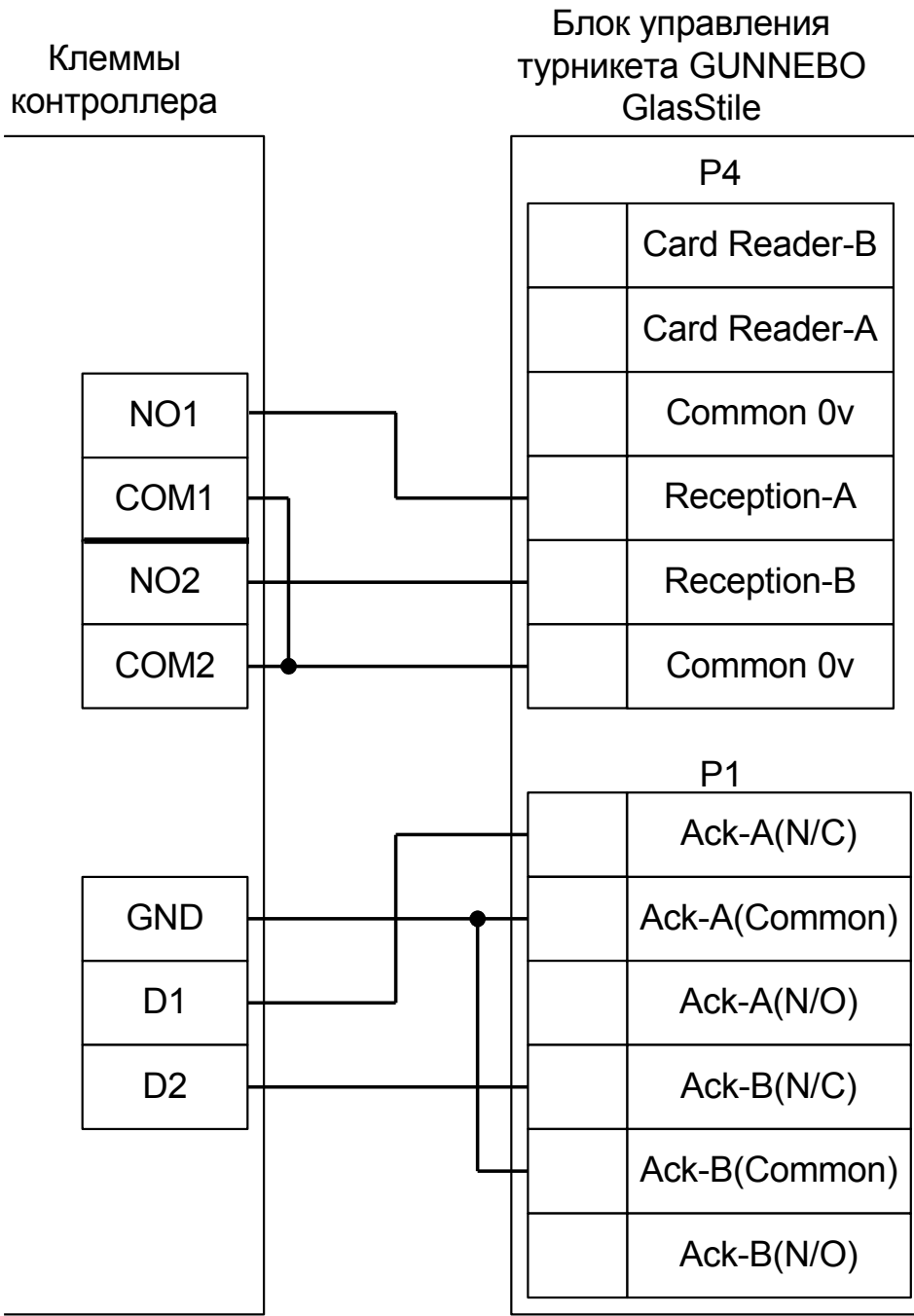
Рисунок 91. Подключение турникета GlasStileNew.
