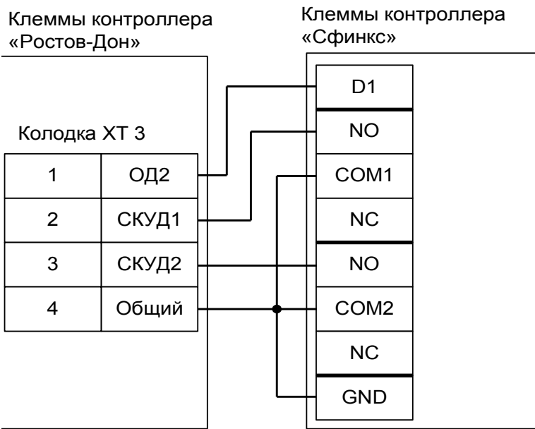
Рисунок 76. Подключение турникетов и калиток «Ростов–Дон», старая электроника, вариант №1.
