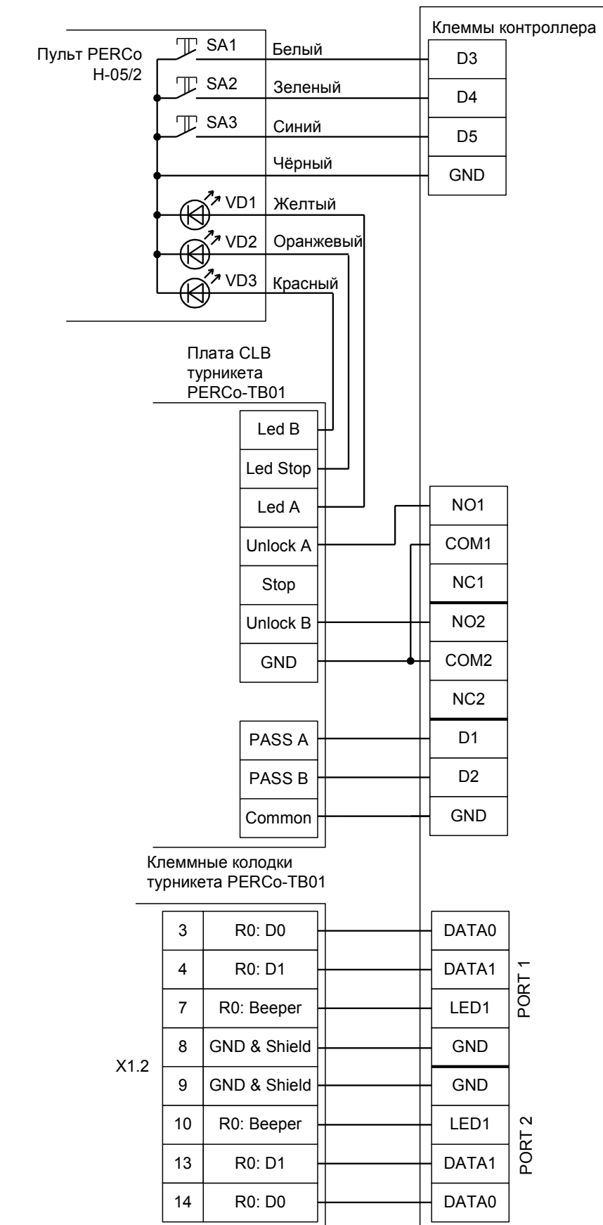
Рисунок 52. Подключение турникета PERCo-TB01.
