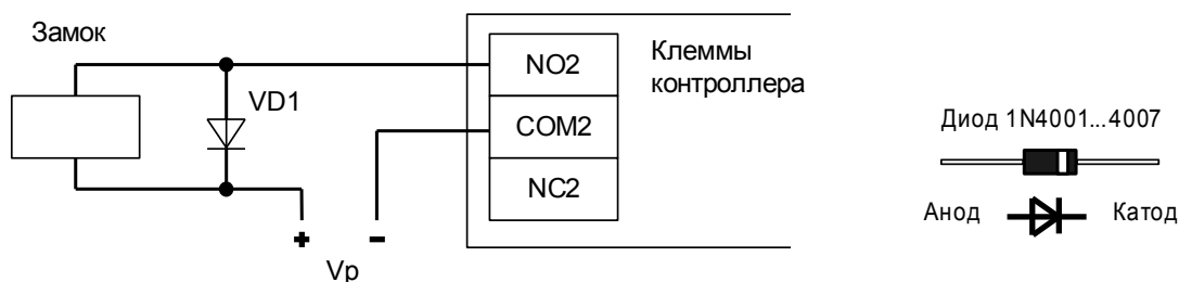
Рисунок 21. Пример подключения электромеханической защёлки, отпираемой напряжением, для первой двери.
