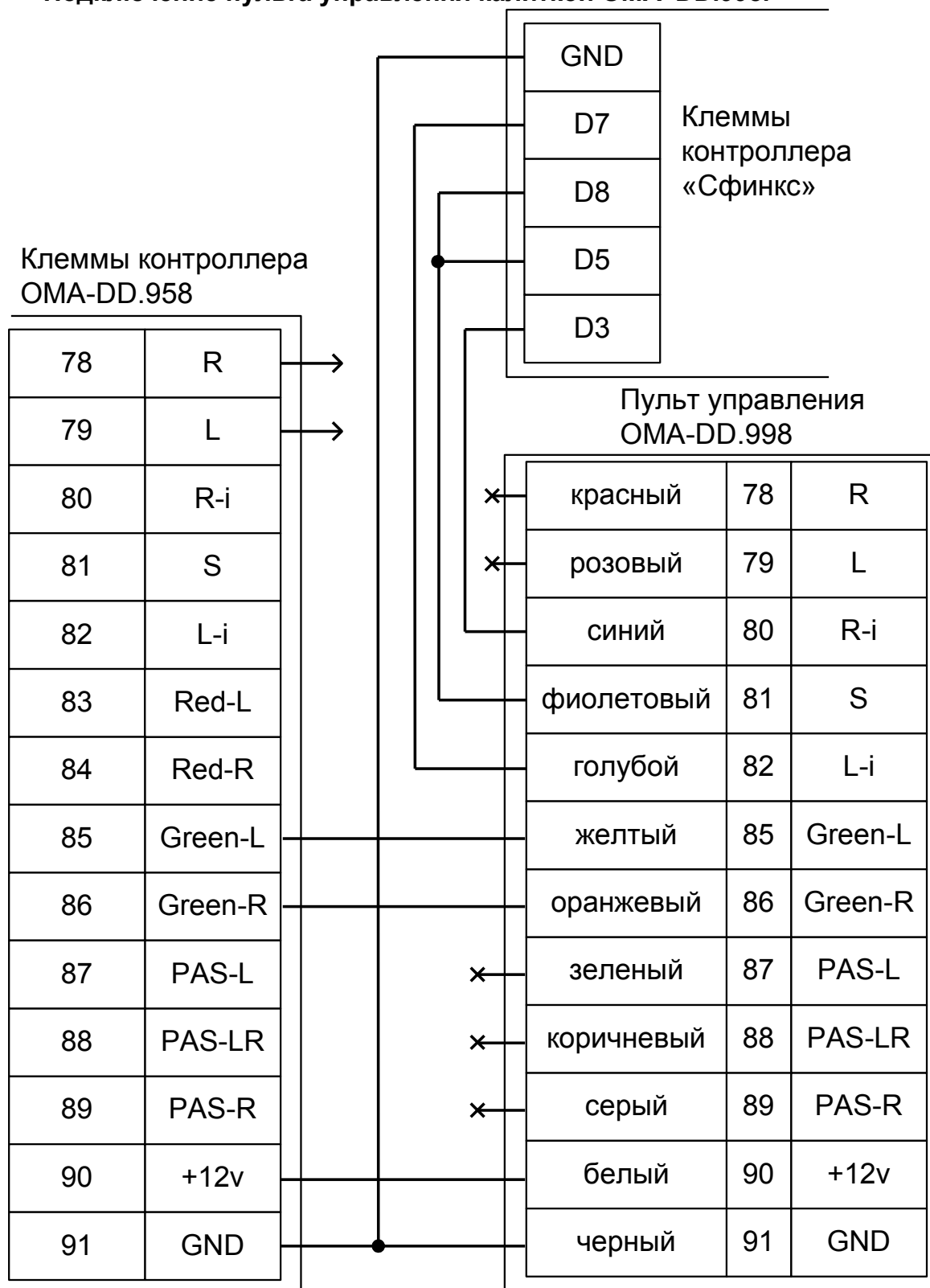
Рисунок 73. Подключение пульта управления калиткой OMA-DD.998.
