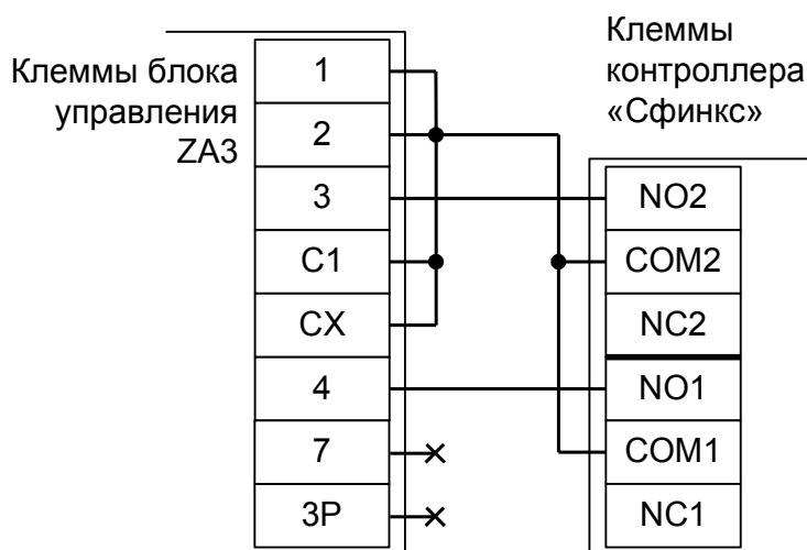
Рисунок 128. Подключение к блоку управления ZA3, ZA3N.
