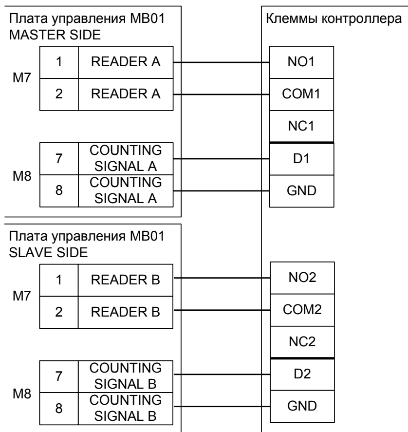
Рисунок 94. Подключение турникетов Gunnebo с платой управления MB01.
