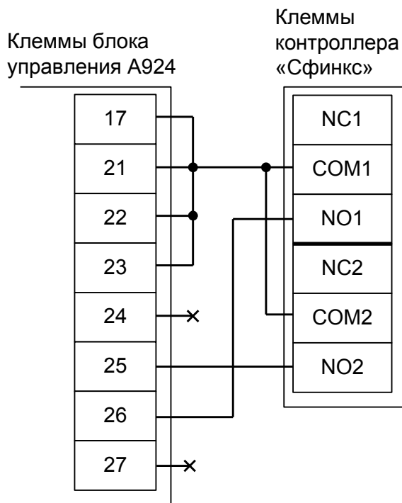
Рисунок 124. Подключение блока управления A924.
