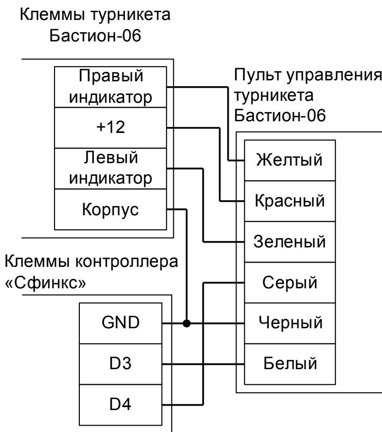
Рисунок 84. Первый вариант подключения пульта управления турникетами «Бастион-06» и «Бизон».
