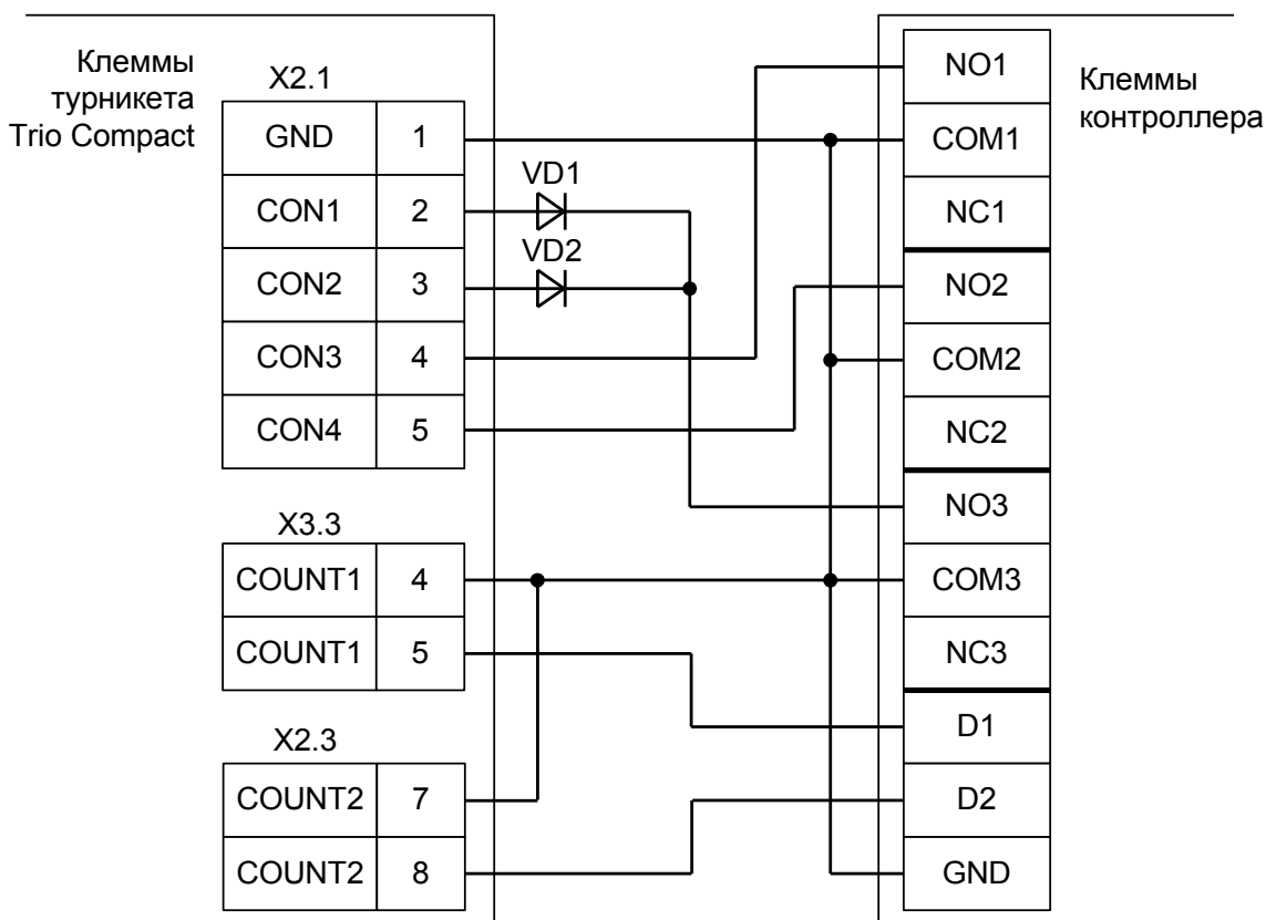
Рисунок 85. Подключение турникета Trio Compact.
