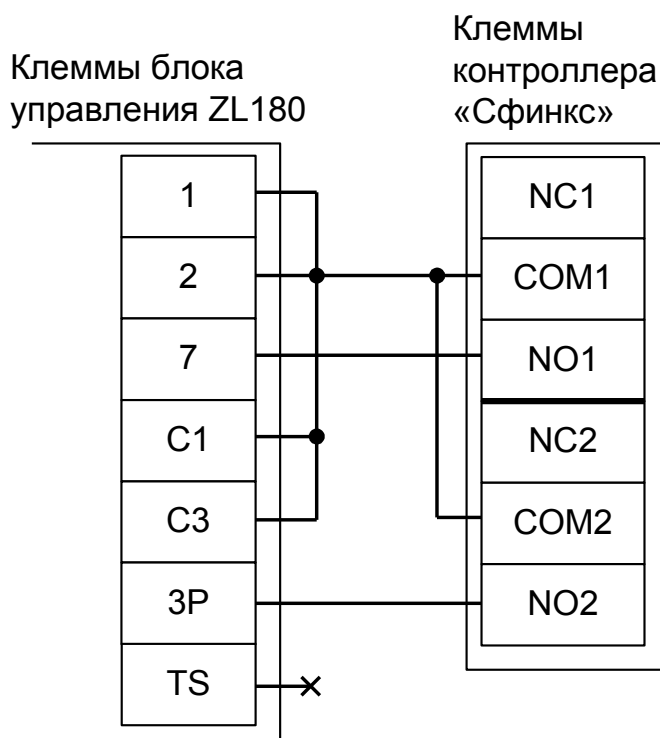
Рисунок 133. Подключение блока управления ZL180.
