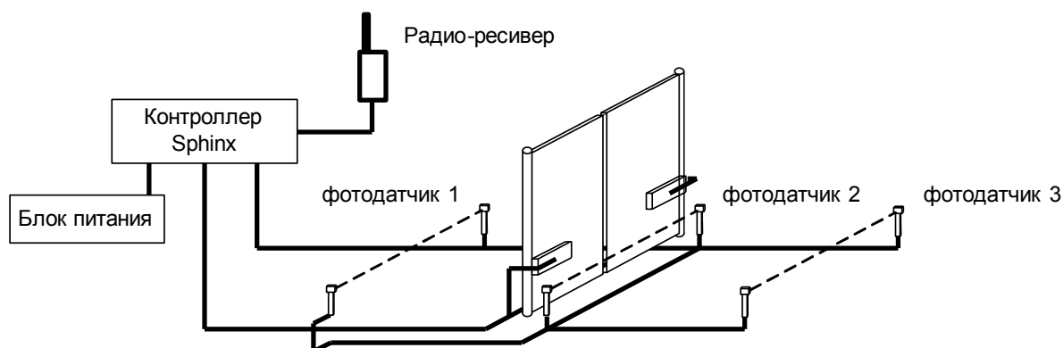
Рисунок 109. Пример автоматизации ворот с использованием радиобрелоков.
