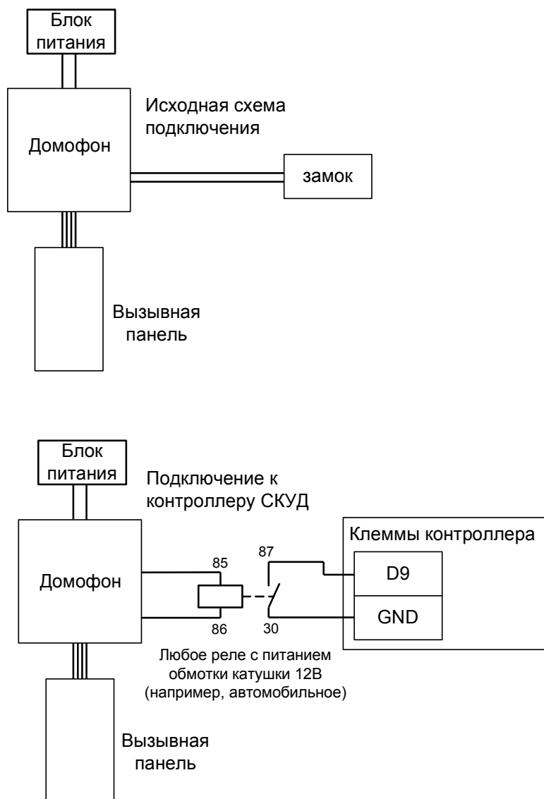
Рисунок 29. Подключение домофона, подающего напряжение непосредственно на замок.
