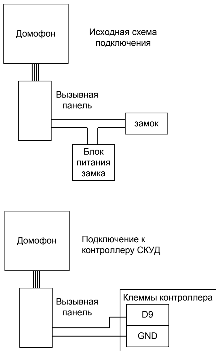
Рисунок 28. Подключение домофона с «сухим контактом» реле.
