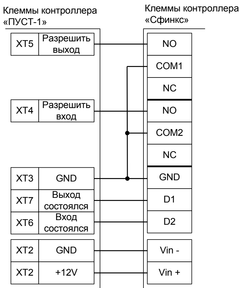
Рисунок 98. Подключение турникета Stella STL-111.
