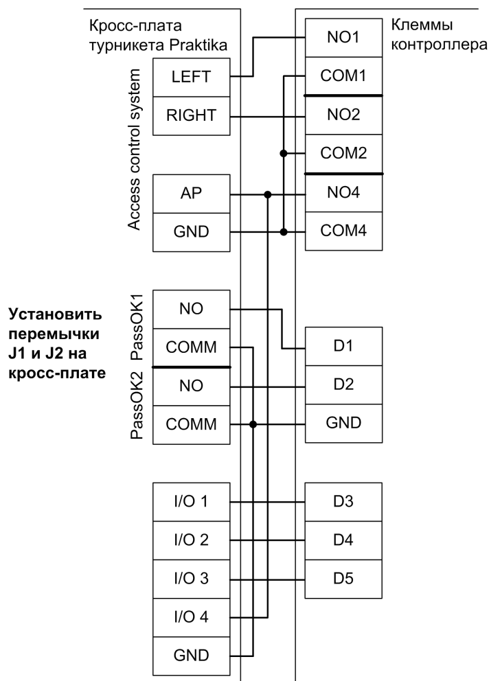
Рисунок 87. Подключение турникетов Praktika.
