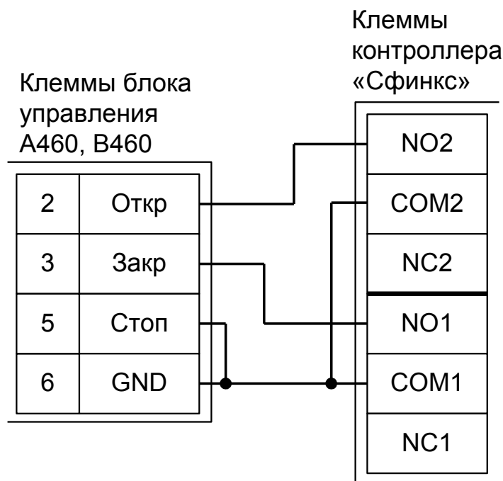
Рисунок 146. Подключение блоков управления Normann A460, B460.
