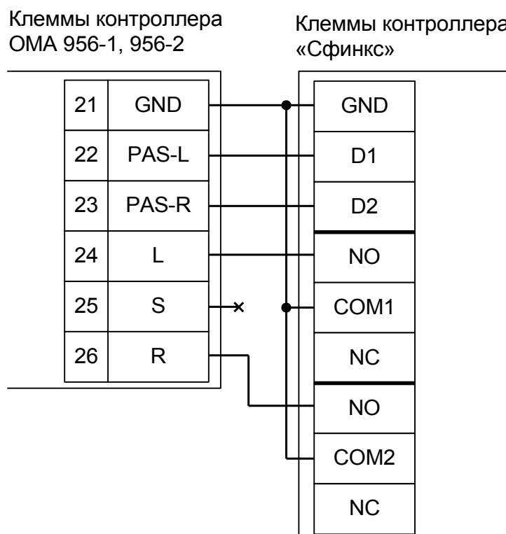
Рисунок 66. Подключение турникета ОМА с контроллером ОМА 956-1, 956-2.
