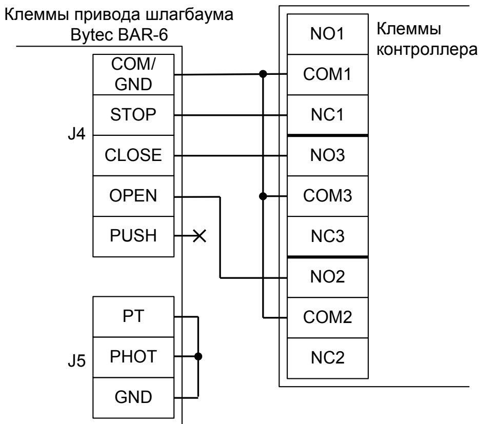
Рисунок 155. Подключение блока управления Bytec BAR-6.
