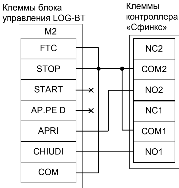
Рисунок 147. Подключение блока управления LOG-BT.
