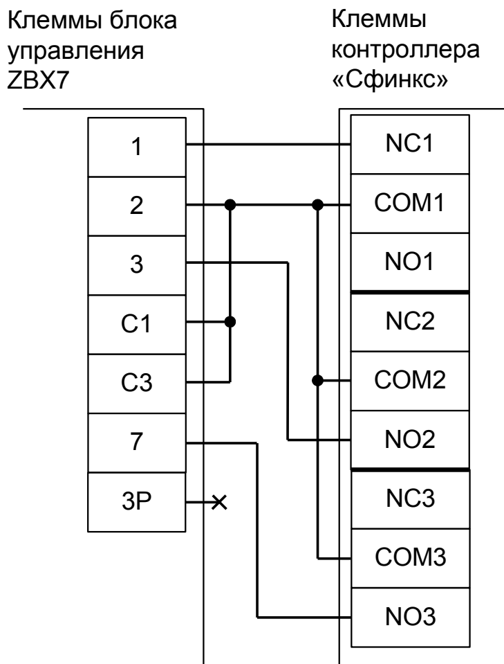
Рисунок 130. Подключение к блоку управления ZBX7.
