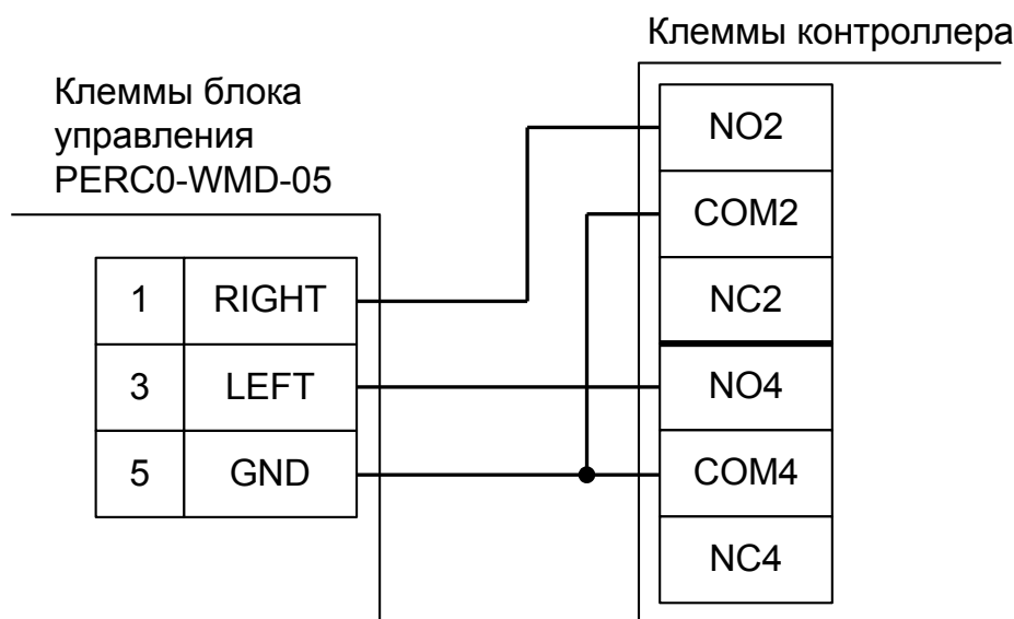
Рисунок 59. Подключение калитки PERCo-WMD-05.
