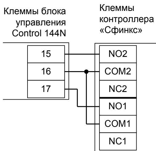
Рисунок 149. Подключение блока управления Control 144N.
