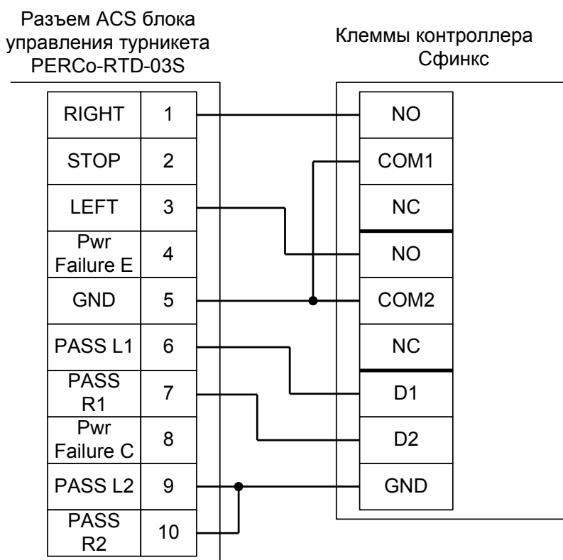
Рисунок 48. Подключение турникета PERCo-RTD-03S.
