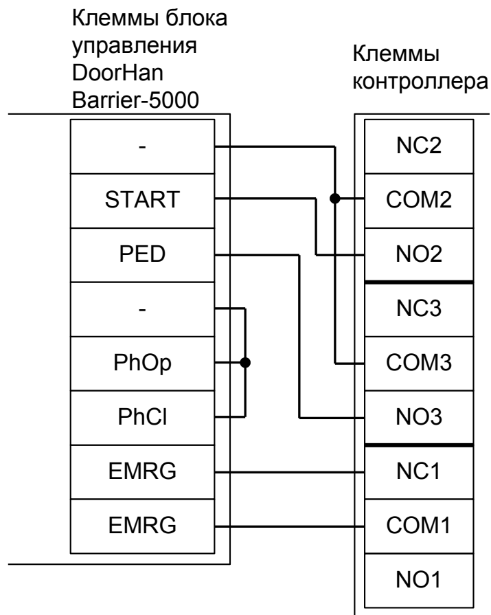
Рисунок 148. Подключение блока управления DoorHan Barrier-5000.
