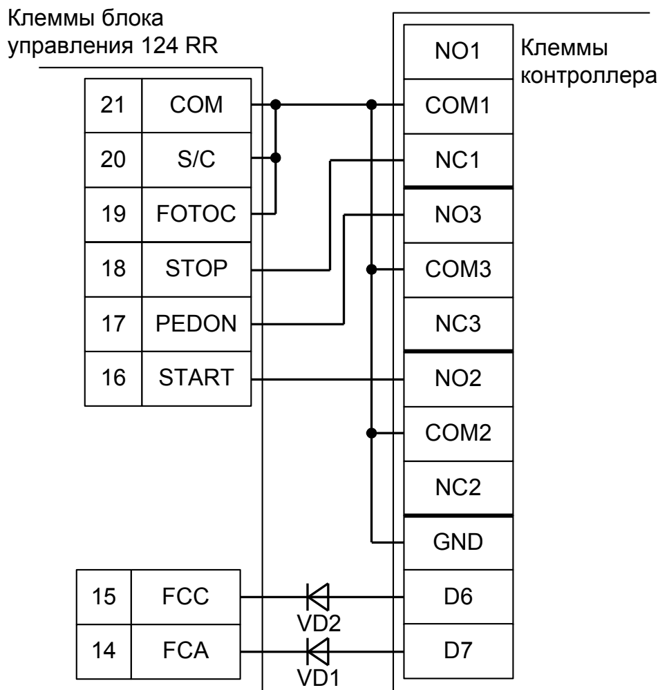
Рисунок 151. Подключение блока управления DEA 124RR.
