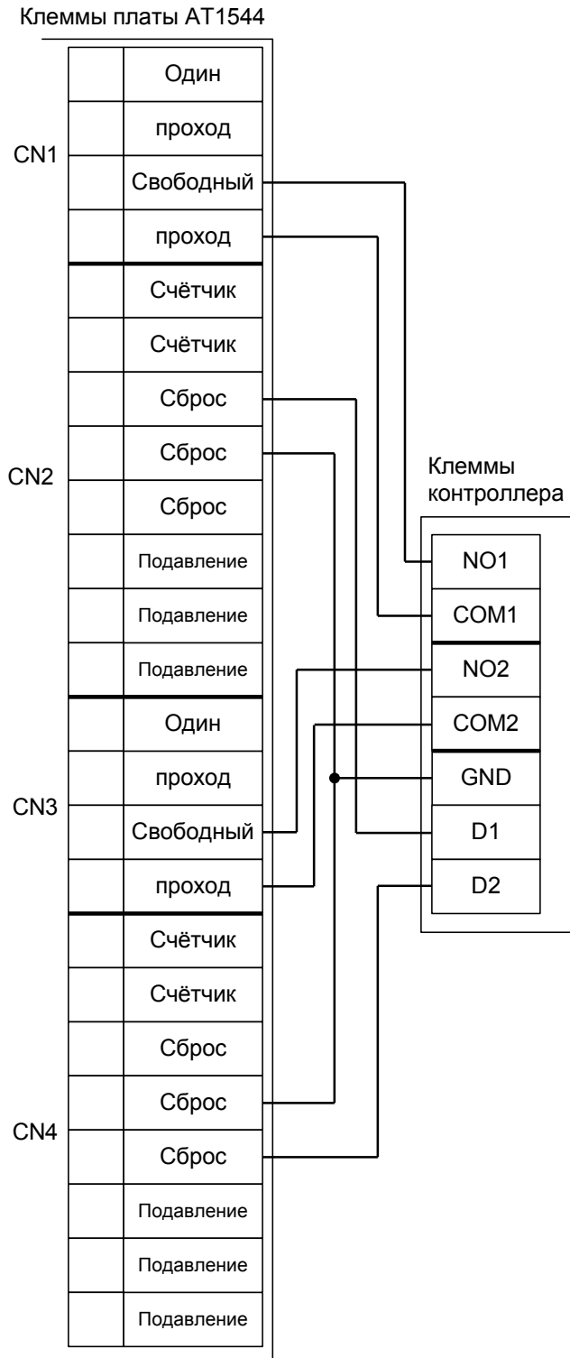
Рисунок 96. Подключение турникетов GUNNEBO RotaSec.
