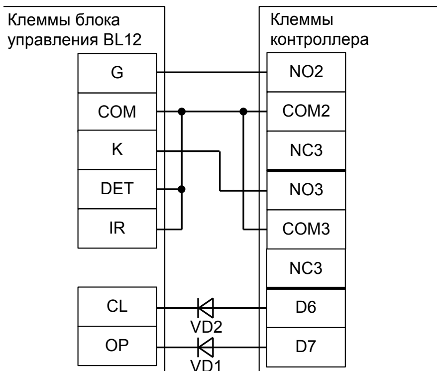
Рисунок 153. Подключение блока управления BL12 с использованием концевых датчиков.
