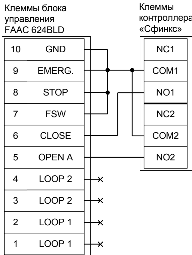
Рисунок 120. Подключение блока управления FAAC 624BLD.
