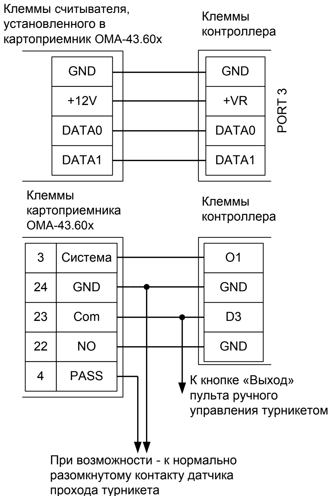
Рисунок 33. Пример подключения картоприёмника ОМА-43.60х в направлении «выход».
