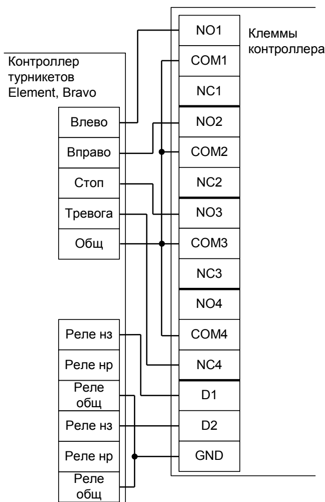
Рисунок 106. Подключение турникетов Element и Bravo.
