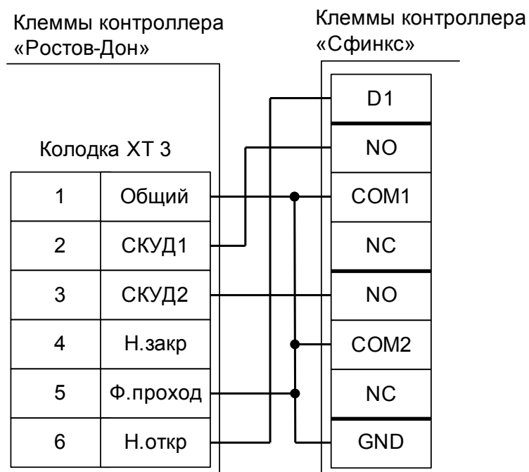
Рисунок 79. Подключение турникетов и калиток «Ростов–Дон», старая электроника, вариант №4.
