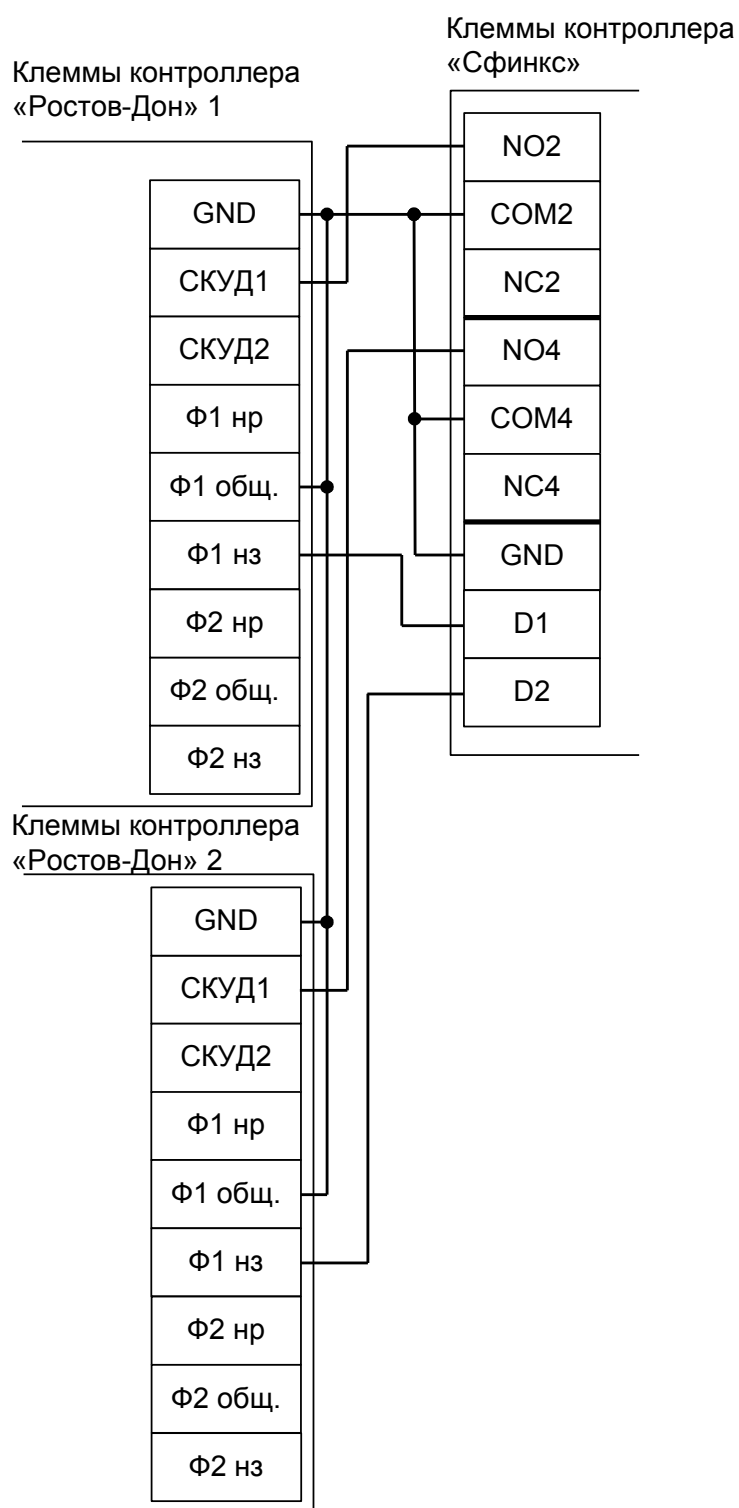
Рисунок 82. Подключение двухпроходного турникета Ростов-Дон.
