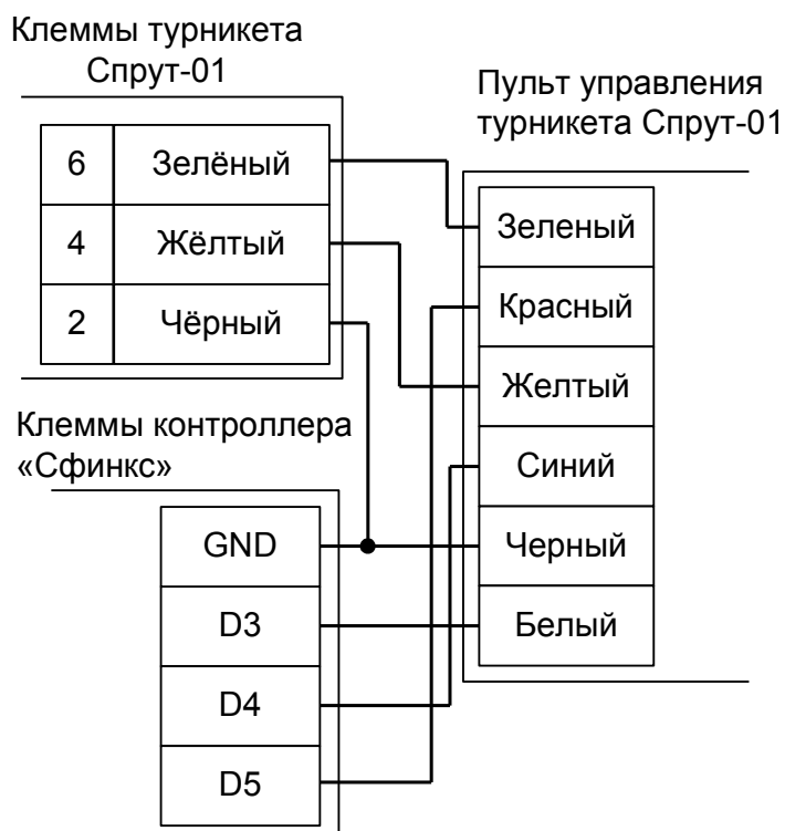
Рисунок 102. Первый вариант подключения пульта управления турникета «Спрут-01».
