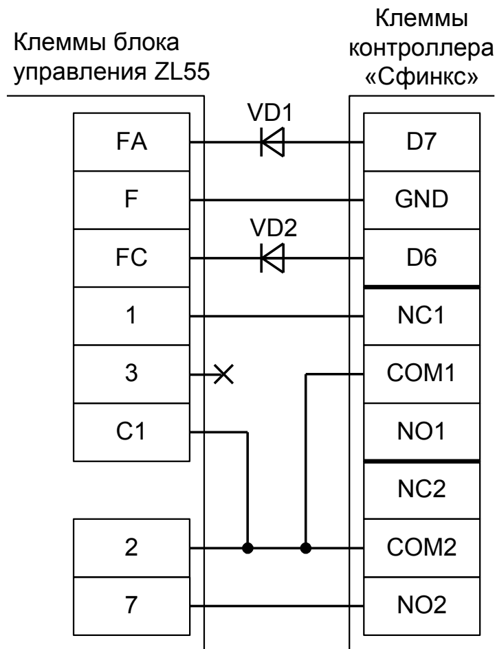
Рисунок 132. Подключение блока управления ZL55 ворот V600, V700.
