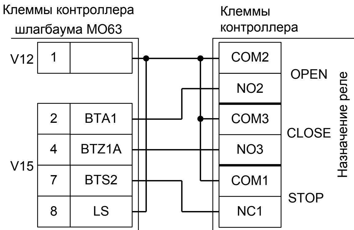
Рисунок 158. Подключение ELKA ES-25M – ES80M.
