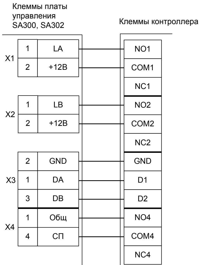
Рисунок 105. Подключение турникетов SA300, SA302.
