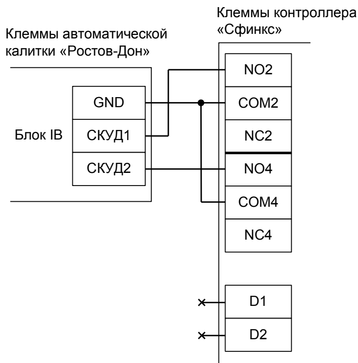
Рисунок 81. Подключение автоматической калитки Ростов-Дон.
