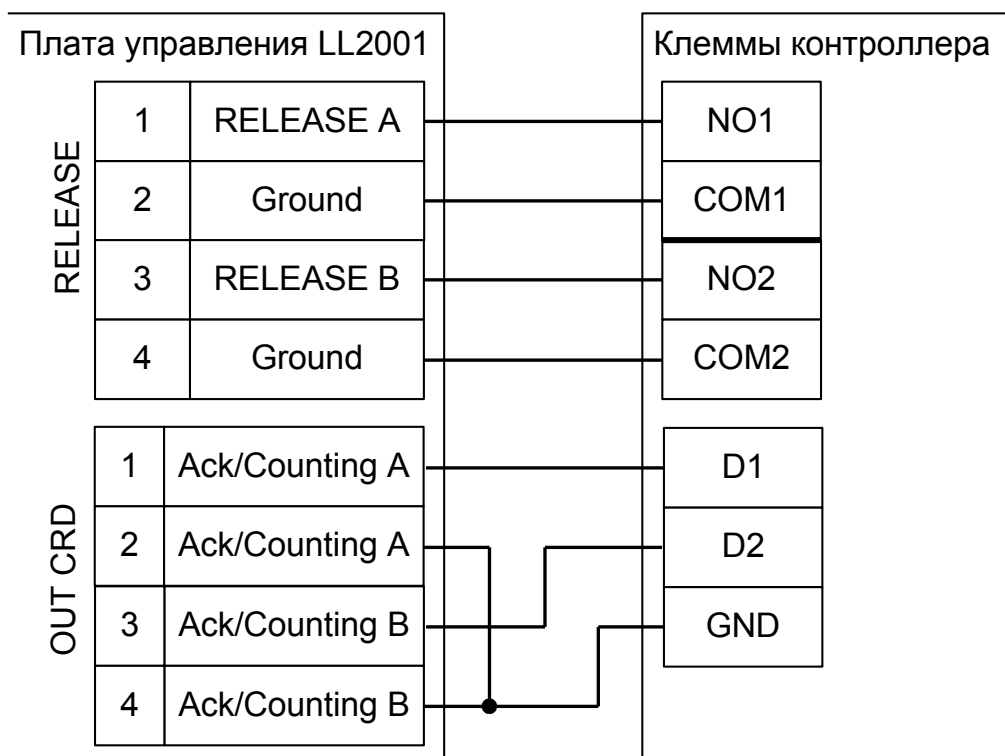
Рисунок 95. Подключение турникетов Gunnebo с платой управления LL2001.
