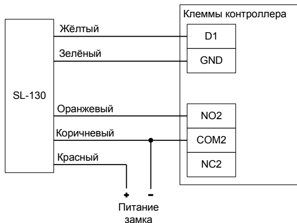
Рисунок 24. Пример подключения замка SL-130 для первой двери.
