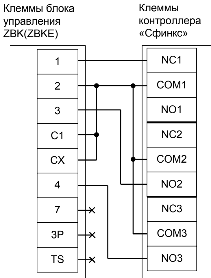
Рисунок 129. Подключение к блоку управления ZBK(ZBKE).
