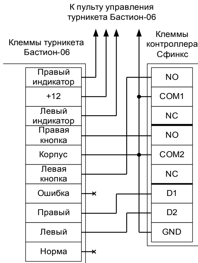
Рисунок 83. Подключение турникетов «Бастион-06» и «Бизон».
