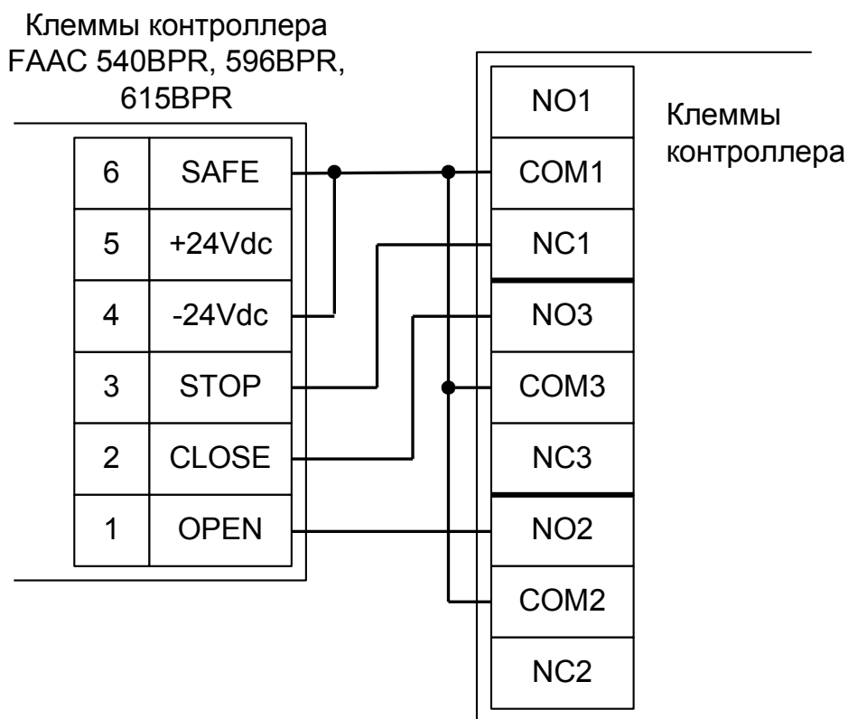
Рисунок 117. Подключение блоков управления FAAC 540BPR, 596BPR, 615BPR.
