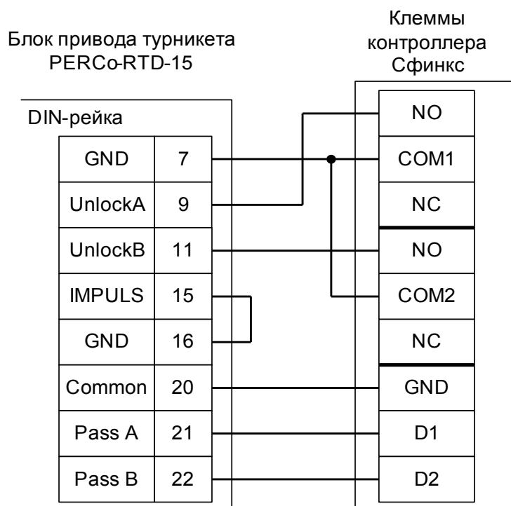
Рисунок 49. Подключение турникета PERCo-RTD-15.
