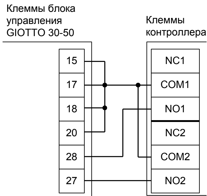
Рисунок 138. Подключение шлагбаумов BFT Giotto 30-50.
