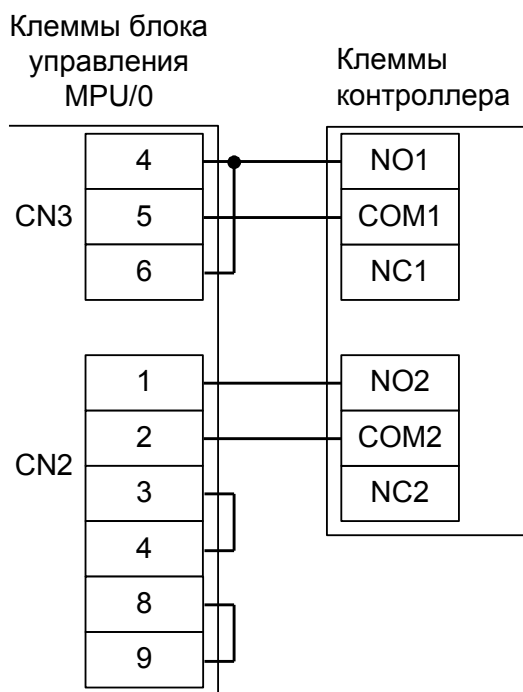
Рисунок 154. Подключение блока управления MPU/0.
