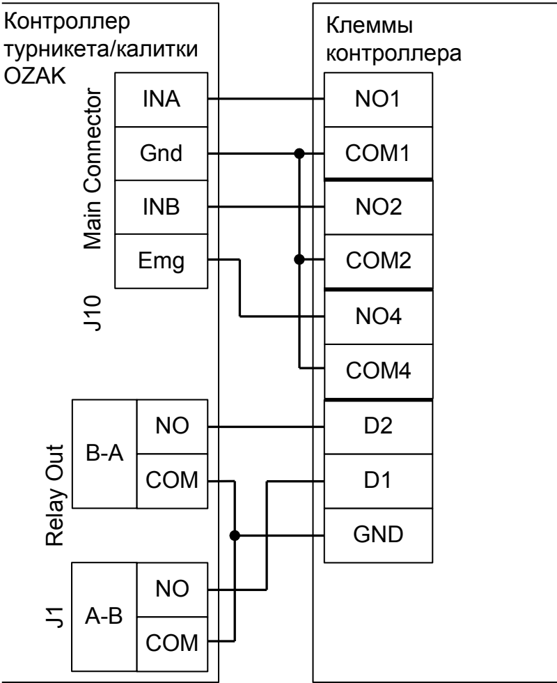
Рисунок 108. Подключение турникетов и калиток OZAK.
