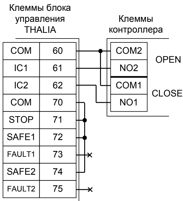
Рисунок 139. Подключение блока управления THALIA.
