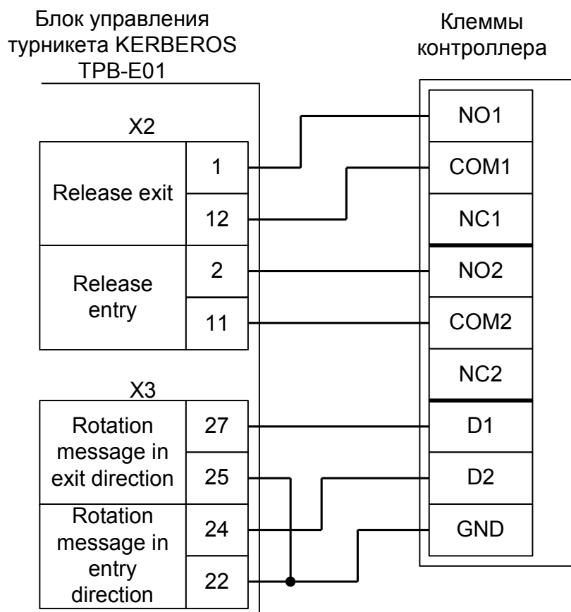
Рисунок 103. Подключение турникетов КАВА Kerberos TPB-E01 с платой управления SINA 2.0.
