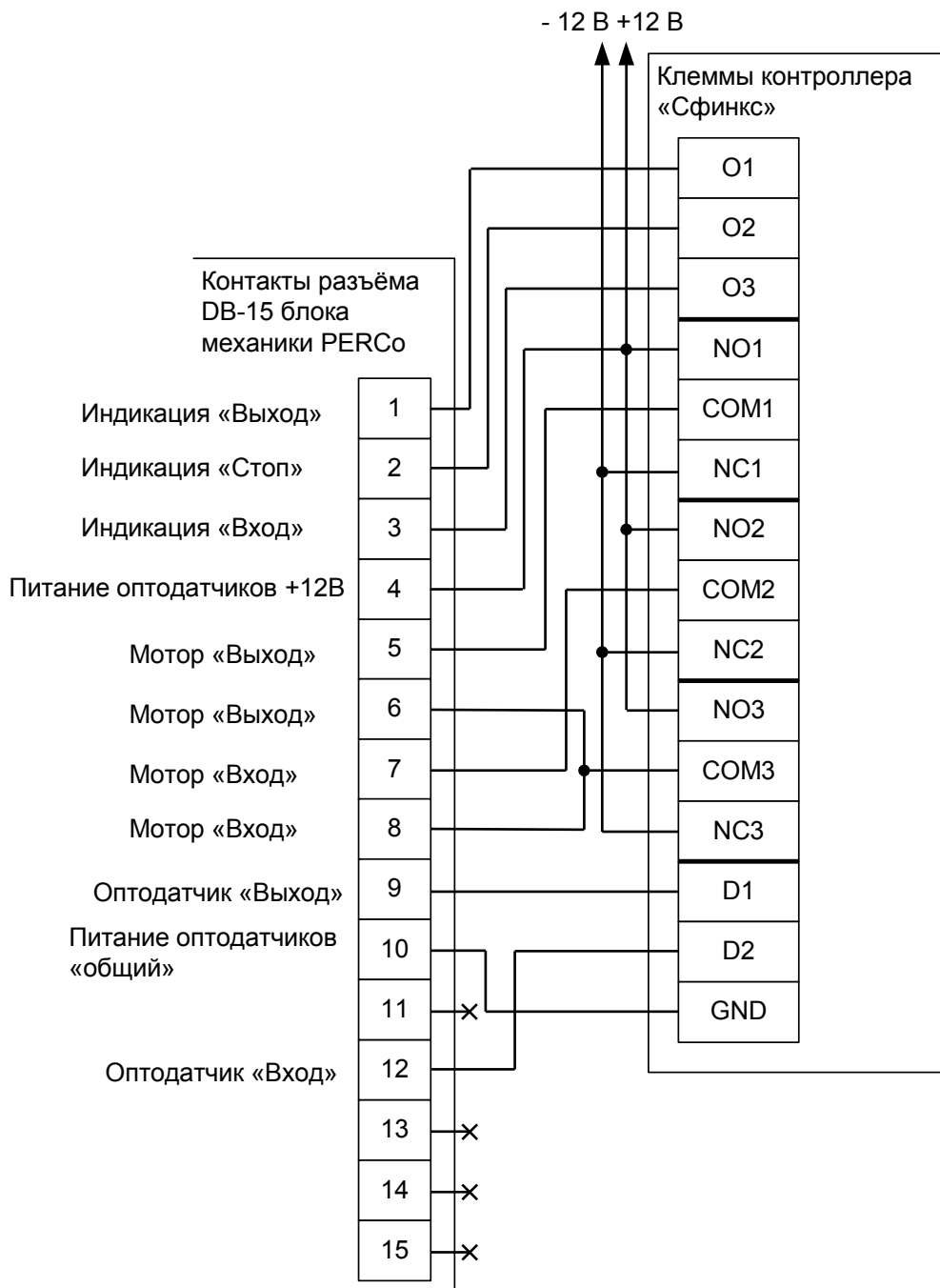
Рисунок 57. Подключение стойки турникета PERCo T-04.
