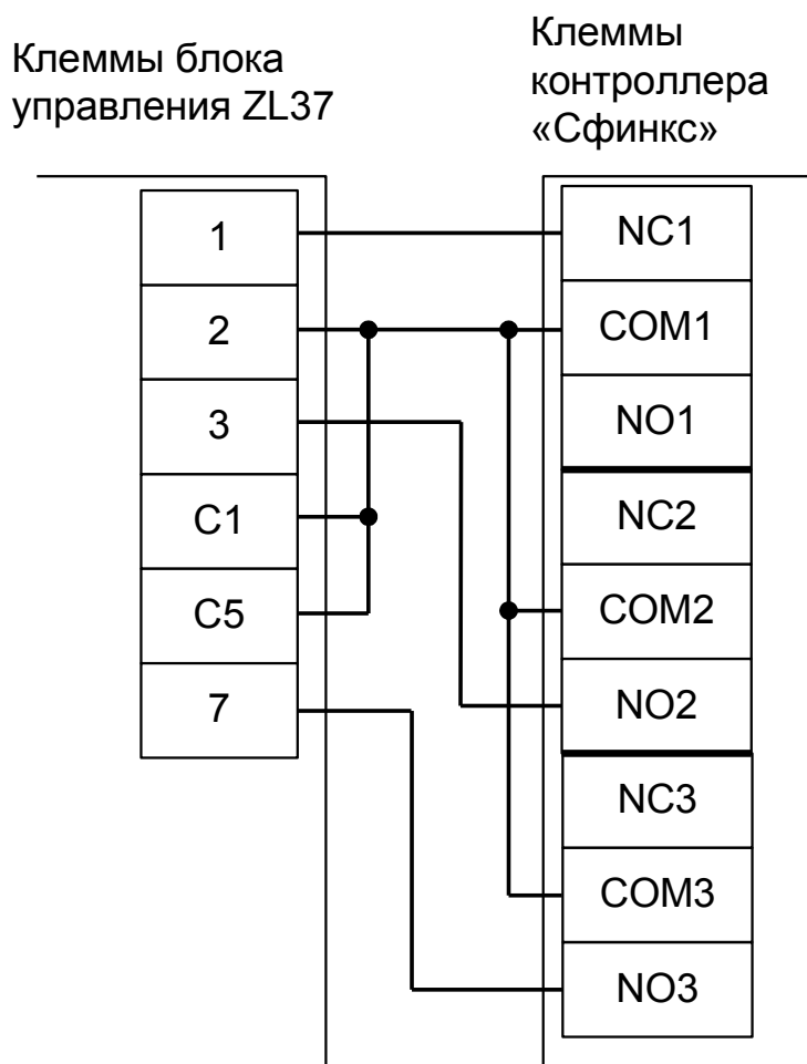
Рисунок 125. Подключение к блоку управления ZL37, ZL38.
