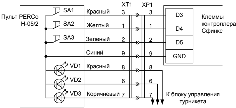
Рисунок 61. Подключение пульта управления PERCo H-05/2 с разъёмом
