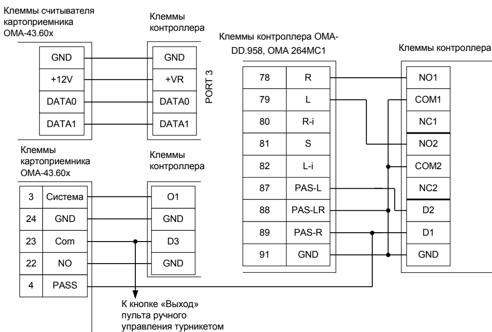
Рисунок 67. Подключение турникета ОМА 26.868.
