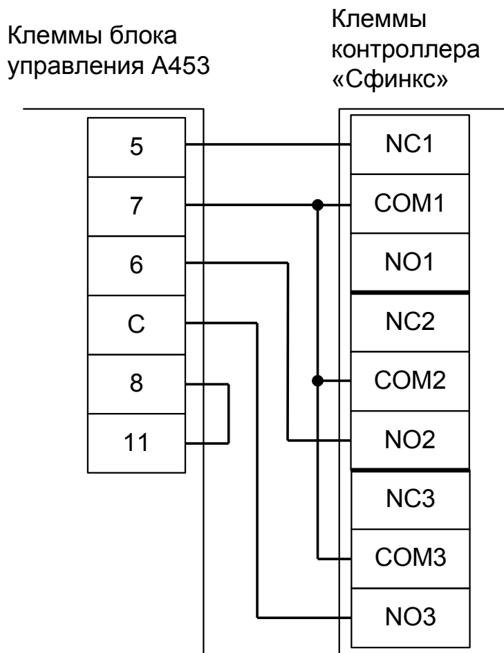
Рисунок 140. Подключение к блоку управления A453.
