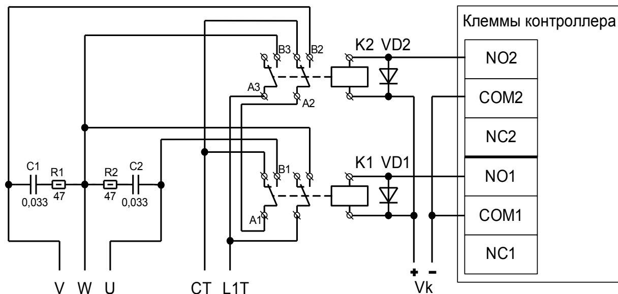
Рисунок 115. Пример подключения к приводу ворот FAST, KRONO, ATI, FERNI для прямого управления моторами.
