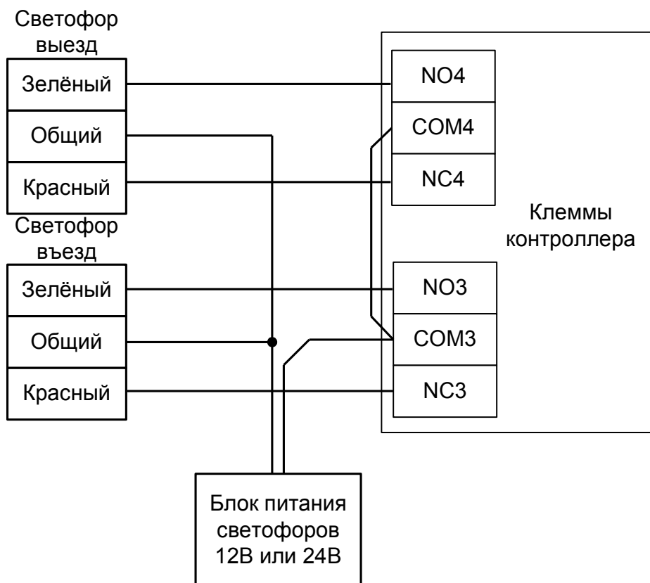
Рисунок 114. Пример подключения светофоров.
