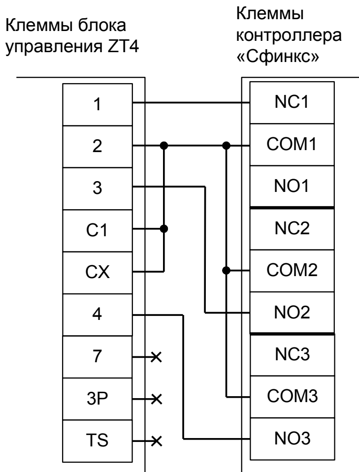
Рисунок 126. Подключение к блоку управления ZT4.
