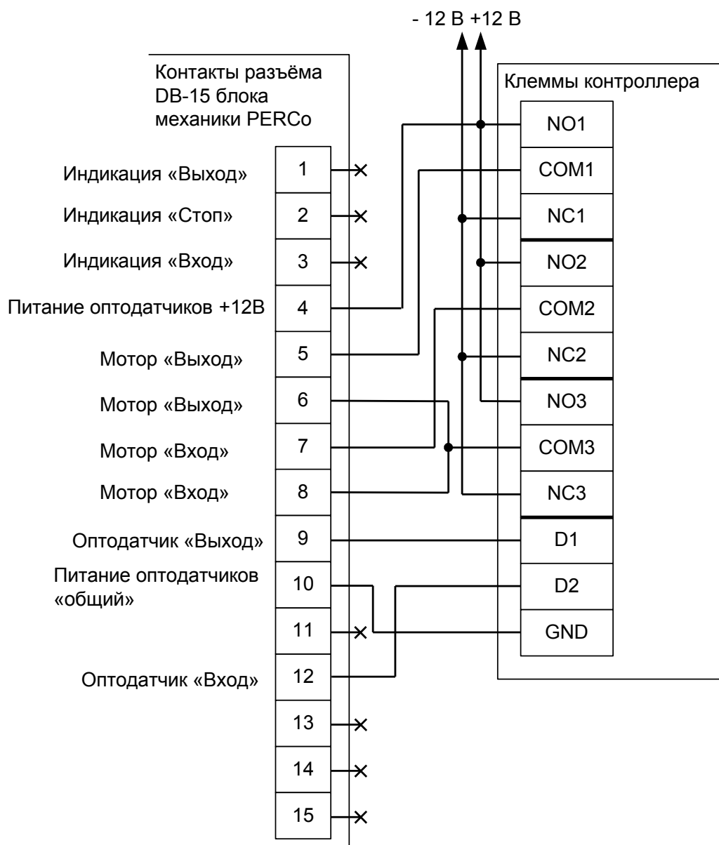
Рисунок 56. Подключение проходных PERCo-КТ02 и КТ05.3.
