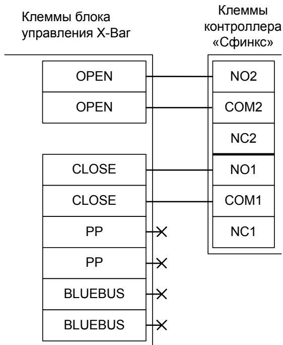
Рисунок 123. Подключение блока управления шлагбаумов X-Bar и приводов ROBUS.
