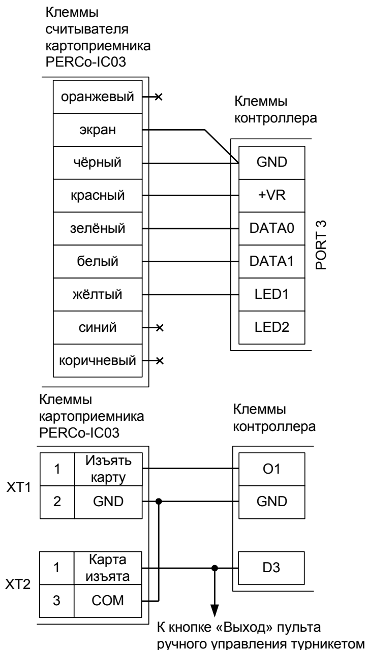
Рисунок 38. Пример подключения картоприёмника PERCo-IC03.
