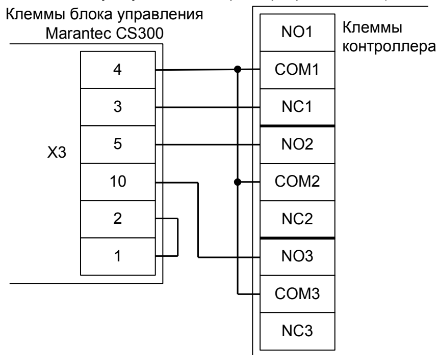
Рисунок 156. Подключение блока управления CS300.
