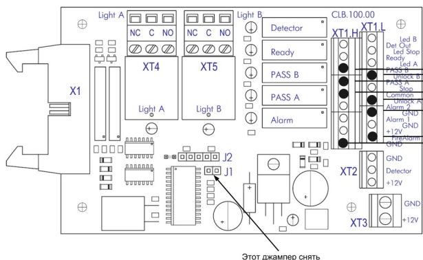
Рисунок 55. Расположение перемычки J1.
