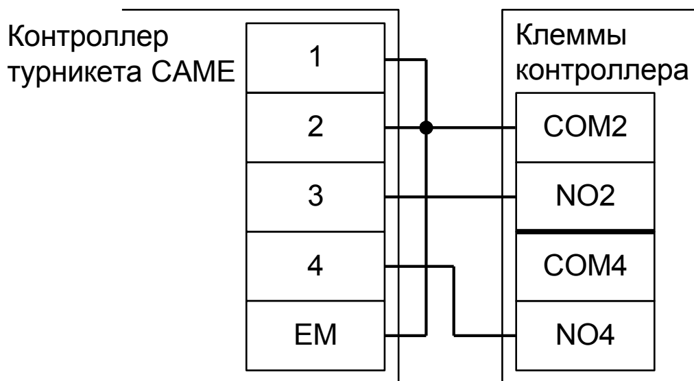
Рисунок 107. Подключение турникета CAME.
