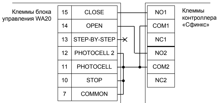
Рисунок 121. Подключение блока управления шлагбаумов WIL4, WIL6.
