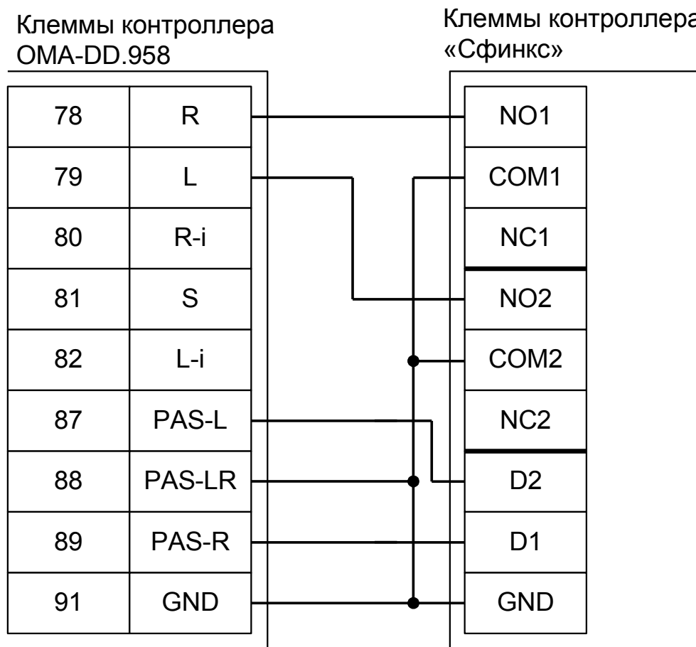
Рисунок 62. Подключение турникета ОМА с контроллером ОМА-DD.958, ОМА 264МС1.
