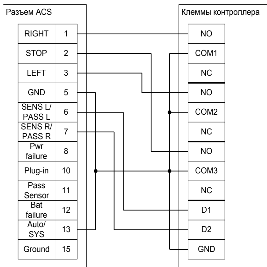
Рисунок 58. Подключение калитки PERCo WHD-04.
