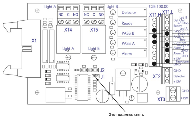
Рисунок 46. Расположение перемычки J1.
