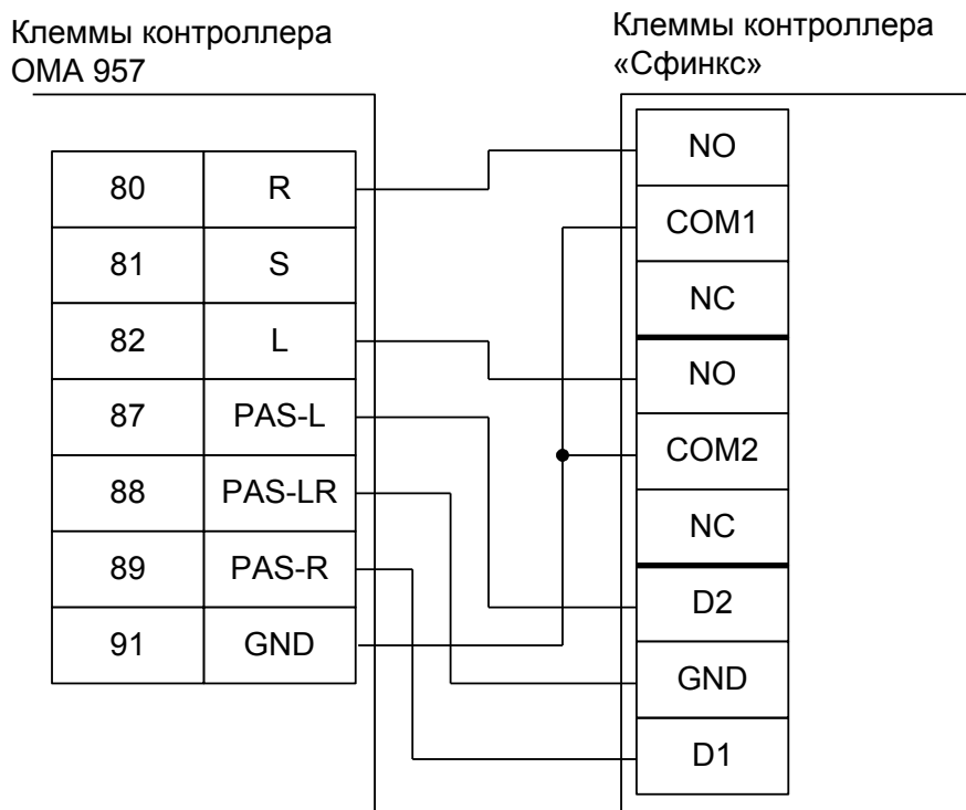
Рисунок 64. Подключение турникета ОМА с контроллером ОМА 957.
