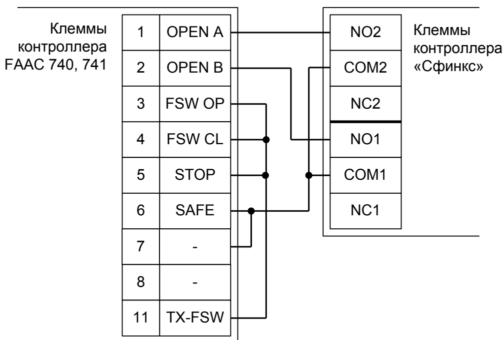
Рисунок 119. Подключение блока управления ворот FAAC 740, 741.
