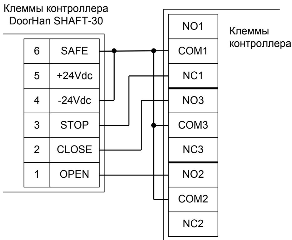
Рисунок 150. Подключение блоков управления DoorHan SHAFT-30.
